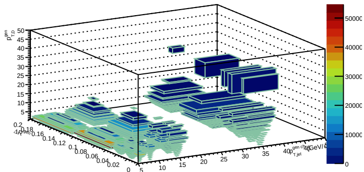
POWHEG + PYTHIA
