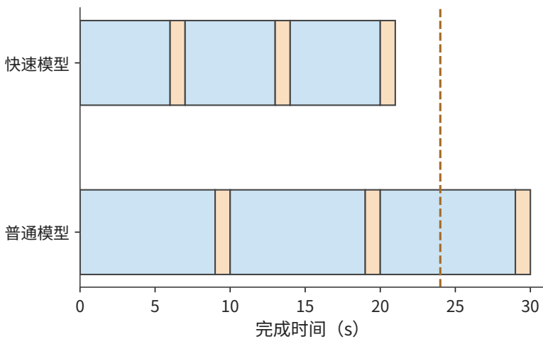
图 11-40：两种方案均在模型调用期间准备环境，工具执行均为每轮 1 秒。模型调用从每轮 9 秒降至 6 秒，三轮结束时刻从第 30 秒移到第 21 秒，从 24 秒期限之后提前到期限之内。
