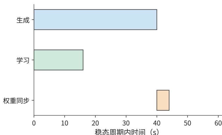
图 10-42：稳态中生成下一批与学习上一批在独立资源上重叠；两者完成后同步权重，周期为 44 s。橙色同步阶段阻塞两侧。
