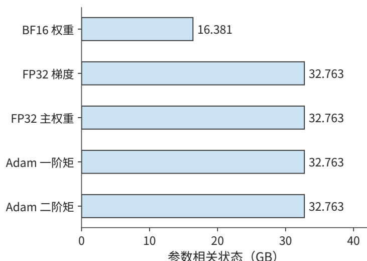
图 3-22 Qwen3-8B 全参数训练的参数相关状态。每参数包括 2 字节计算权重和 4 组 4 字节状态，共 18 字节；激活和工作区的容量需求按各自的生命周期单独计算。
