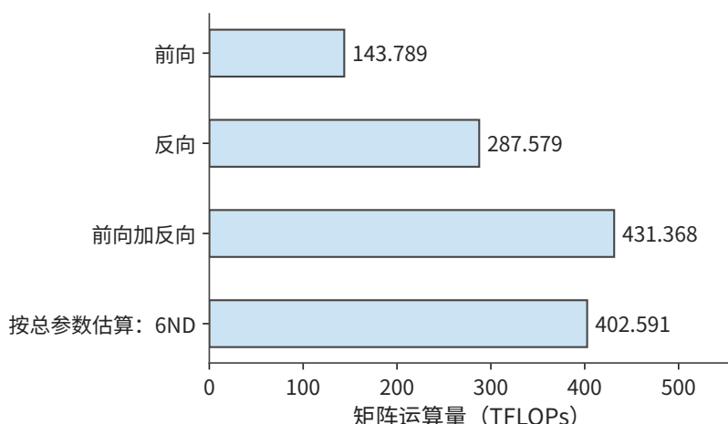
图 3-23 Qwen3-8B、8192 个 token 输入的全参数训练。全部输入 token 执行词表头、没有重计算；按矩阵逐项累计，前向加反向为 431.368 TFLOPs。
