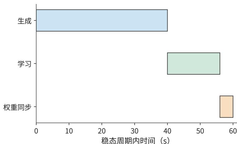
图 10-41：同步循环依次生成本批样本、学习本批样本、同步权重，分别用时 40、16、4 s，共 60 s。
