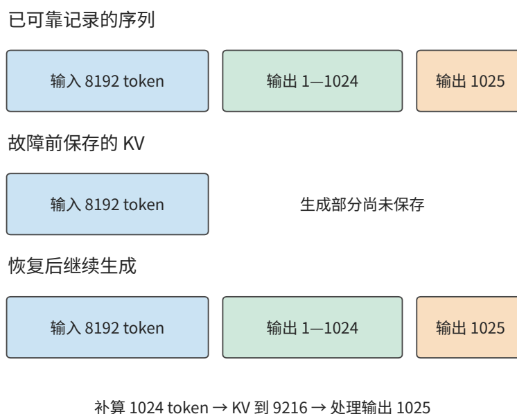
图 9-44：输出记录决定继续哪条序列，KV checkpoint 决定从哪里补算。假定 1025 个输出均已可靠记录，但 KV 只保存了原输入。下方按输入、前 1024 个输出和第 1025 个输出分段示意，宽度不按 token 数量比例绘制。
