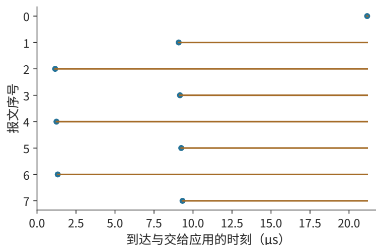
图 7-47：序号 0 丢失后按算例等待时间重传，其他七个报文保留在接收方。只补发缺失报文后，约 21.2 \mu\text{s} 全部可交付。圆点表示报文到达，横线表示到达后等待缺口补齐的时间，纵轴是报文序号。
