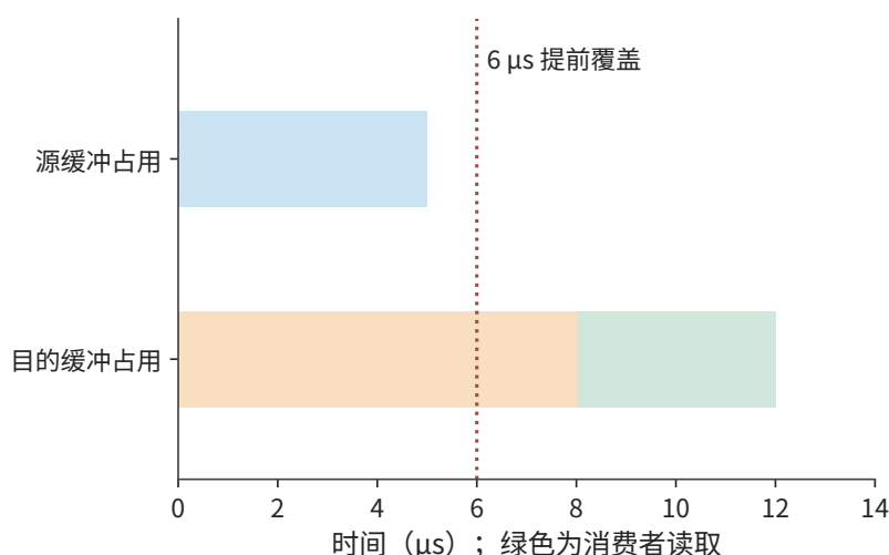
图 7-30：源缓冲占用到 5 μs 发送完成；目的缓冲持续占用到 12 μs 消费者用完。绿色为 8–12 μs 的读取区间。虚线标出 6 μs 提前覆盖目的地址的错误操作。
