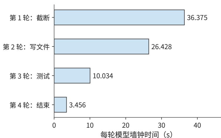
图 3-10 代码任务中四轮模型调用的实际耗时，各轮从自己的起点计时。模型时间合计 76.294 秒，工具合计约 0.078 秒，整任务另含控制与交接时间。
