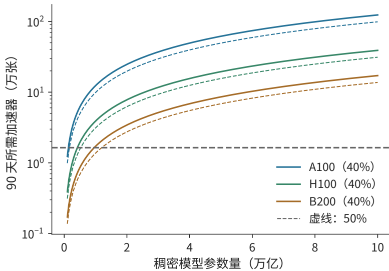
图 10-46：固定 90 天执行期限，稠密模型规模增大要求更多的卡。数据量为 20T token，算法工作为 6ND ，实线的 MFU 为 40%，虚线为 50%，使用 BF16 稠密矩阵峰值。各线为向上取整前的连续计算边界；横线标出 16,384 张卡。
