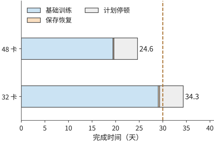
图 10-44：每条横条依次累计基础训练时间、保存与故障恢复的附加时间，以及预留的 5 天计划性停顿。基础训练时间已经包括通信和输入等待；橙色小段为 checkpoint 模型得到的额外耗时。两套方案使用相同任务和全局 batch，虚线标出 30 天期限。
