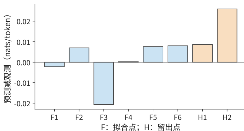
图 3-27 同一组预测误差的放大视图。F1—F6 为拟合点，H1—H2 为留出点；纵轴是预测减观测，保留正负号。
