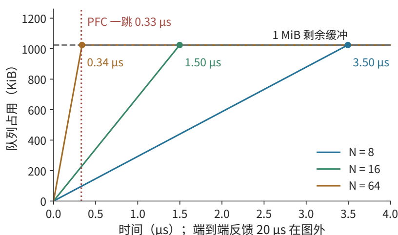
图 7-44： N = 8、16、64 时队列以 300、700、3100 \text{ GB/s} 的超额速率增长，圆点标出 1 \text{ MiB} 剩余缓冲被填满的时刻 3.50、1.50、0.34 \mu\text{s} 。竖直虚线是 PFC 的一跳反馈距离 0.33 \mu\text{s} ，三条线在这之前都没有填满；端到端反馈的 20 \mu\text{s} 在图的横轴之外。
