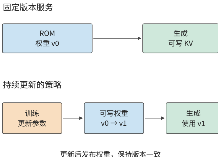
图 10-39：固定版本服务与策略训练的权重生命周期。上方 ROM 重复提供同一版本；下方训练产生新版本并发布给生成端。KV 写入与权重更新使用不同的数据通路。
