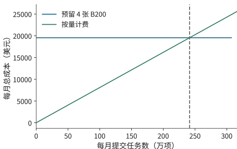
图 11-33：4 张 B200 预留一个月共 19,555.2 美元，按量成本为 0.0081N 美元，N 为提交任务数。两条线在约 241 万项相交，对应预留 GPU 约 78.6% 的利用率；预留线止于每月 307.2 万项的处理上限。
