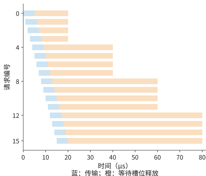
图 7-39：增加槽位后，后续请求更早提交。完成通知仍每 20 μs 批量处理四项，最后一个槽位仍在 80 μs 释放。两图时间轴相同。
