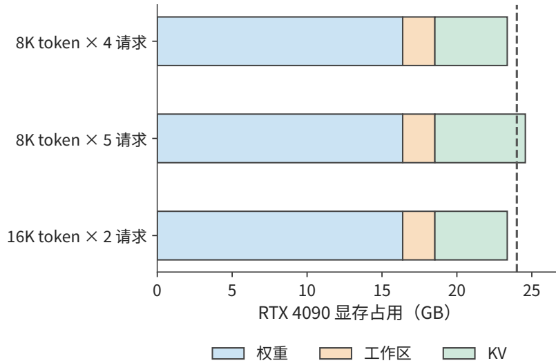
图 4-13 RTX 4090 的 24 GB 显存中的权重、工作区和 KV。8K 四请求与 16K 两请求可以容纳，8K 五请求超过虚线标出的容量上限。
