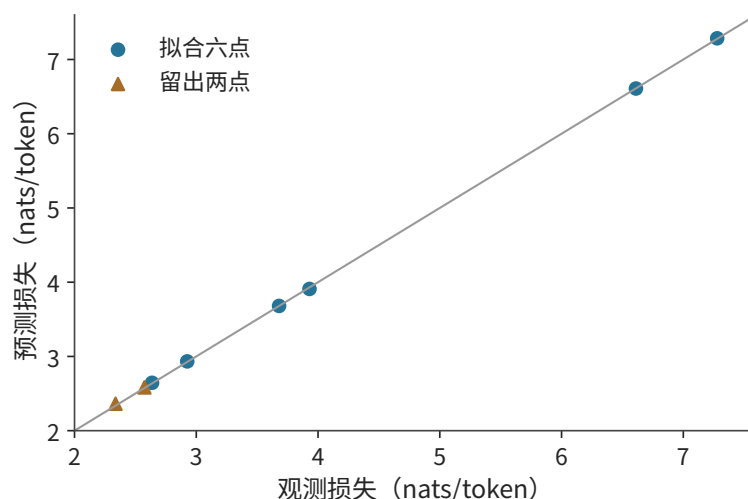
图 3-26 八个公开 C4 观测的预测与实际损失。6 点用于拟合，2 点预先留出作检验；对角线表示预测等于观测，点到线的偏差反映误差。
