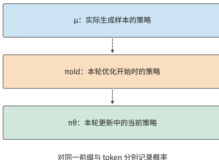
图 10-40: \mu 产生训练样本, \pi_{old} 标识本轮优化的起点, \pi_{\theta} 随本轮更新变化。虚线表示版本演进顺序。三个概率必须针对同一前缀与同一 token 计算。
