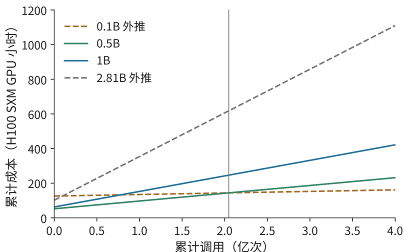
图 3-28 训练与服务累计成本的题设比较。截距是训练投入，斜率是单次调用成本；虚线标出超出拟合参数或数据范围的方案，竖线为约 2.048 亿次的成本交点。图例中的 B 表示十亿个模型参数；纵轴为按 40% MFU 折算的 H100 SXM GPU 小时。
