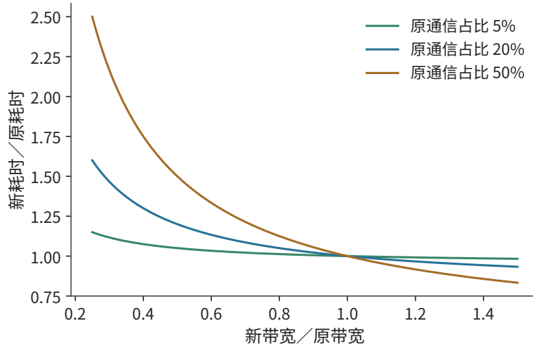
图 10-45：资源能力变化的收益由原有等待时间占比决定。曲线按 T'/T = 1 - f + f/r 计算，固定单卡计算与依赖，通信时间与有效能力成反比。
