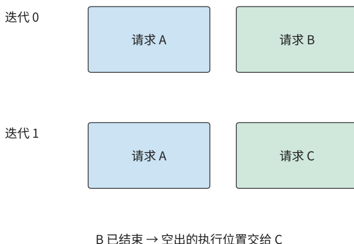
图 8-1: A 跨越两个迭代继续执行。B 在第一轮结束，下一轮由 C 接替其执行位置（每轮为一条活跃请求预留的一行计算）；请求状态仍按各自身份保存。
