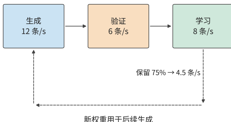
图 10-36：三阶段分别最多处理 12、6、8 条等长轨迹/s。验证后保留 75%，所以只有 4.5 条/s 进入学习。返回箭头表示学习产生的新权重影响后续生成；其同步耗时在后面的阶段切换与异步算例中展开。
