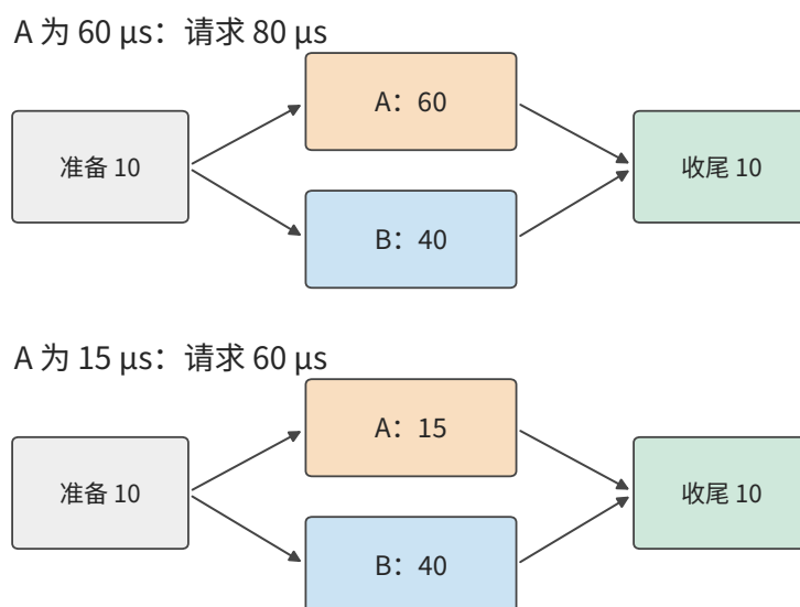
图 5-38: 收尾等待 A、B 两条分支。A 从 60 \mu s 缩短至 15 \mu s 后, 较慢分支由 A 切换为 B, 请求从 80 \mu s 降至 60 \mu s。准备和收尾各为 10 \mu s, 两条分支使用独立资源。
