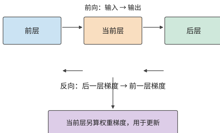
图 3-21 训练沿前向依赖计算输出，再沿反向依赖传递梯度。当前层既向前层传输入梯度，也计算自己的权重梯度，供优化器更新。
