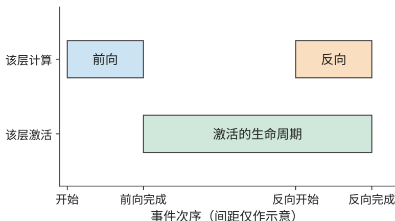
图 3-20 激活的生命周期：一层激活从前向完成后保留到相应反向用完。横轴按事件排列，间距仅表示过程顺序；相应反向计算用完这些激活后，即可释放其占用的空间。
