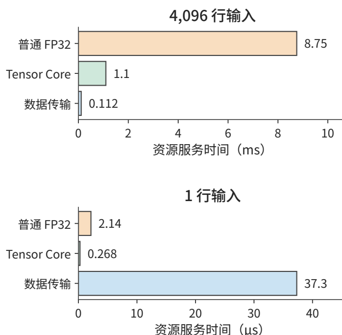
图 4-26 同一 V100 上的 Q 投影。4,096 行时，Tensor Core 大幅缩短矩阵计算；一行时，两条计算路径都短于权重传输。上下两组使用分别标注的时间单位。
