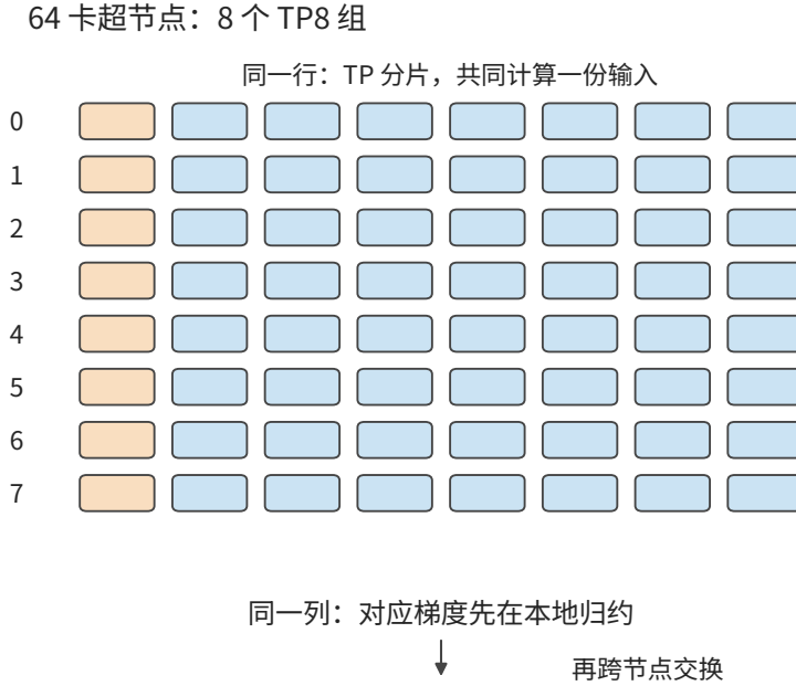
图 7-61：64 卡超节点由八个张量并行组组成。同一行的八张卡处理同一 micro-batch 的不同模型分片；同一列的八张卡先在节点内汇合对应的梯度，再与其他超节点交换同一片。一个训练作业用上全部的卡，不等于全部的卡组成一个张量并行组。
