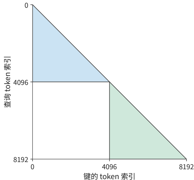
图 10-28：两条 4096 个 token 的序列的因果注意力配对。每个查询 token 读取本序列中不晚于自己的位置，形成两个三角形；两条序列的注意力计算彼此独立，总配对数为 16781312。
