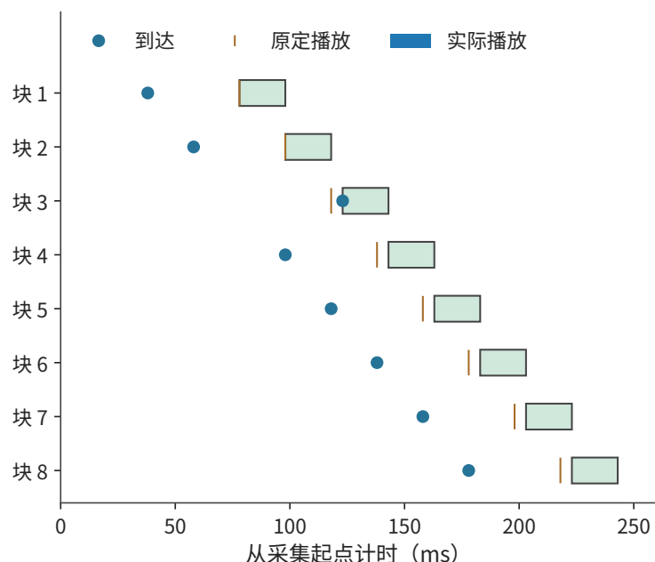
图 3-18 八块音频的教学播放时间线。每块长 20 ms，圆点标到达，短竖线标原定播放时刻，色条标实际播放；第三块晚到 5 ms，后续播放随之顺延。
