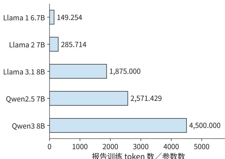
图 3-29 相近参数规模的模型投入不同数量的训练 token。柱值为报告训练数据量除以参数量，Qwen 采用模型系列披露的数据预算。
