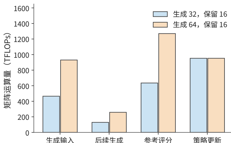
图 3-25 保持 16 条有效样本的目标，生成数由 32 增到 64。生成时的输入处理、后续 decode 和参考模型评分随回答总数增加，策略更新处理的样本数保持相同。
