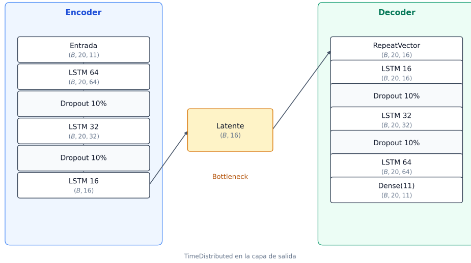
FIGURA 3.4. Arquitectura del autoencoder LSTM: codificador, bottleneck latente y decodificador.
