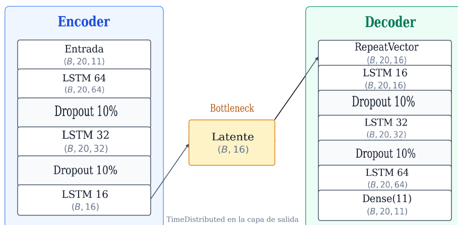
FIGURA 3.4. Arquitectura del autoencoder LSTM: codificador, bottleneck latente y decodificador.
