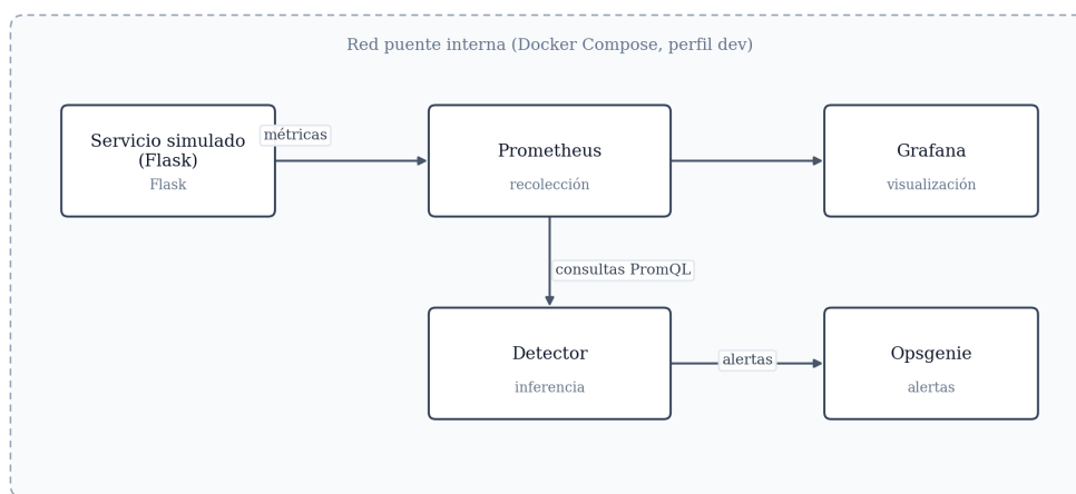
FIGURA 3.2. Topología de despliegue del sistema de detección.
