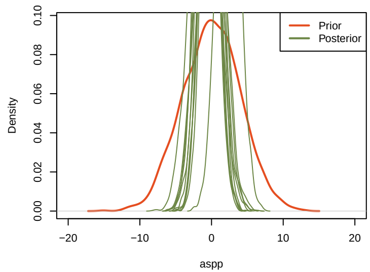
priorVSposterior_aspp
