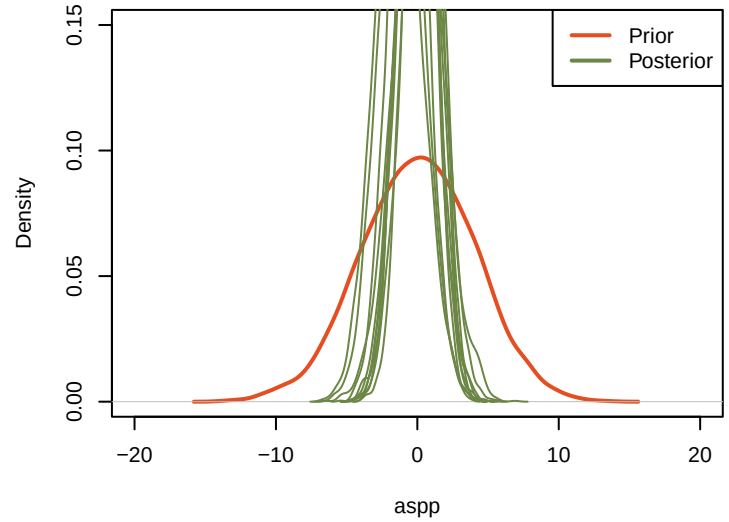
priorVSposterior_aspp
