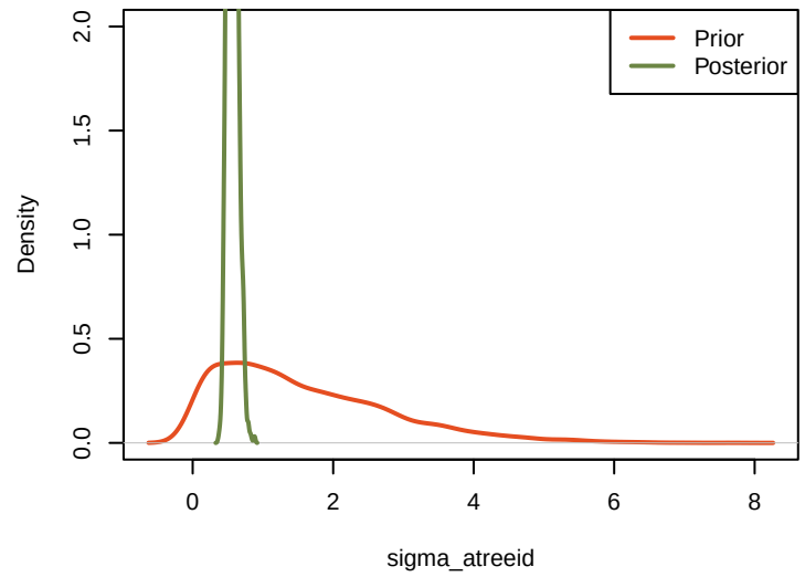
priorVSposterior_sigma_atreeid
