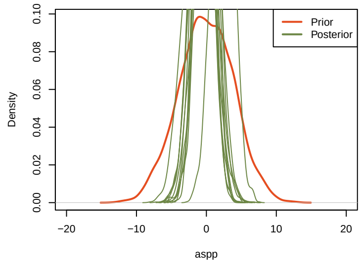
priorVSposterior_aspp
