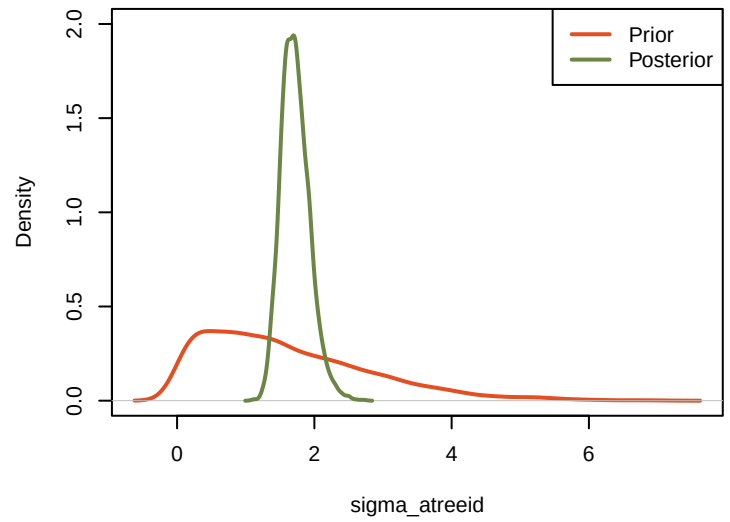
priorVSposterior_sigma_atreid
