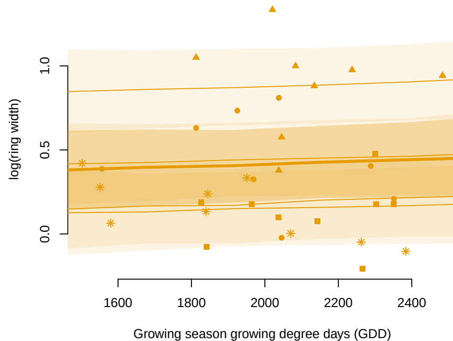
P. deltooides
