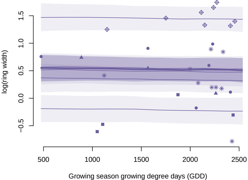
Ae. flava
