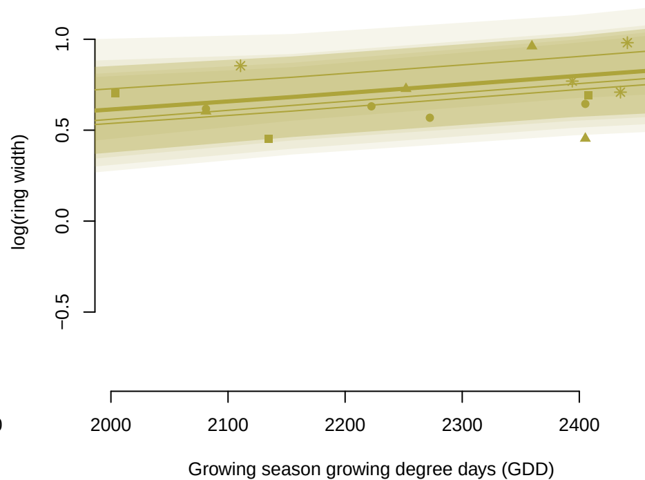
Q. rubra
