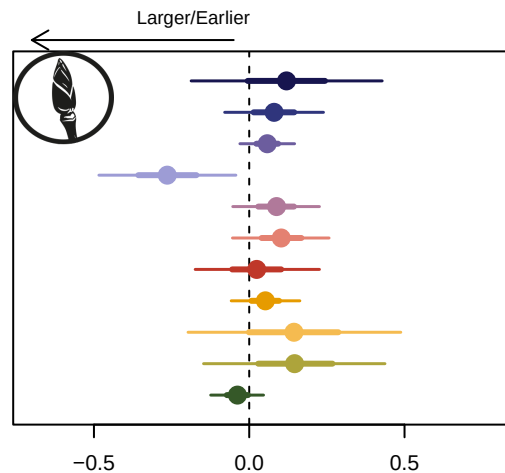
(d) End of season
