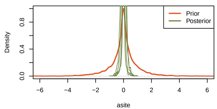
priorVSposterior_asite
