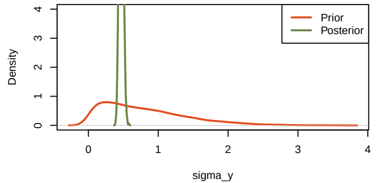
priorVSposterior_sigma_y
