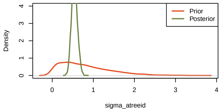
priorVSposterior_sigma_atreeid
