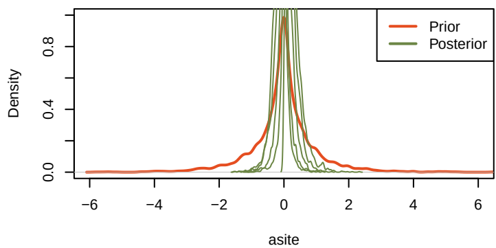
priorVSposterior_asite
