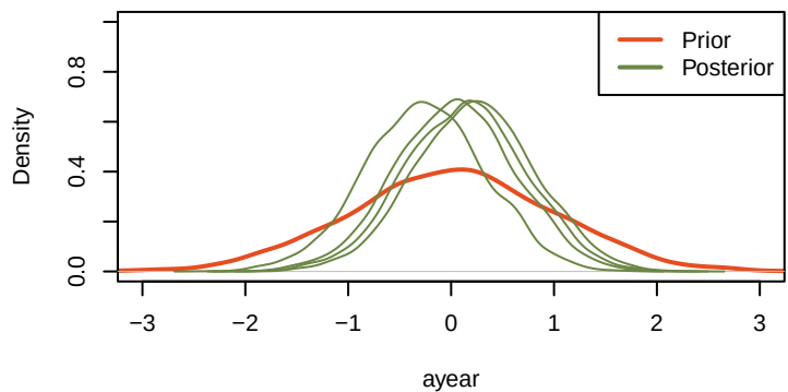
priorVSposterior_ayear
