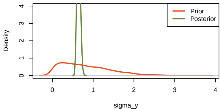
priorVSposterior_sigma_y
