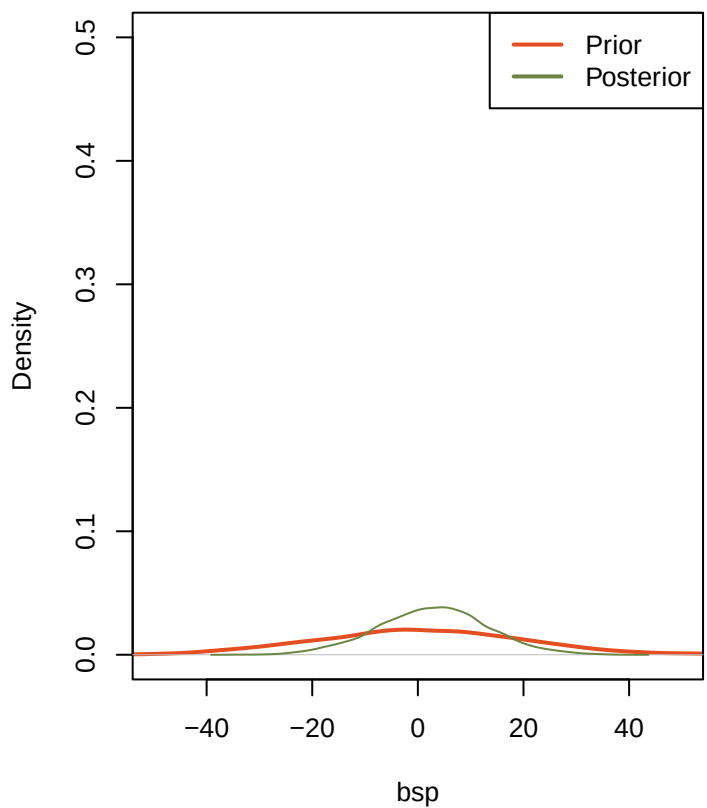
priorVSposterior_bsp
