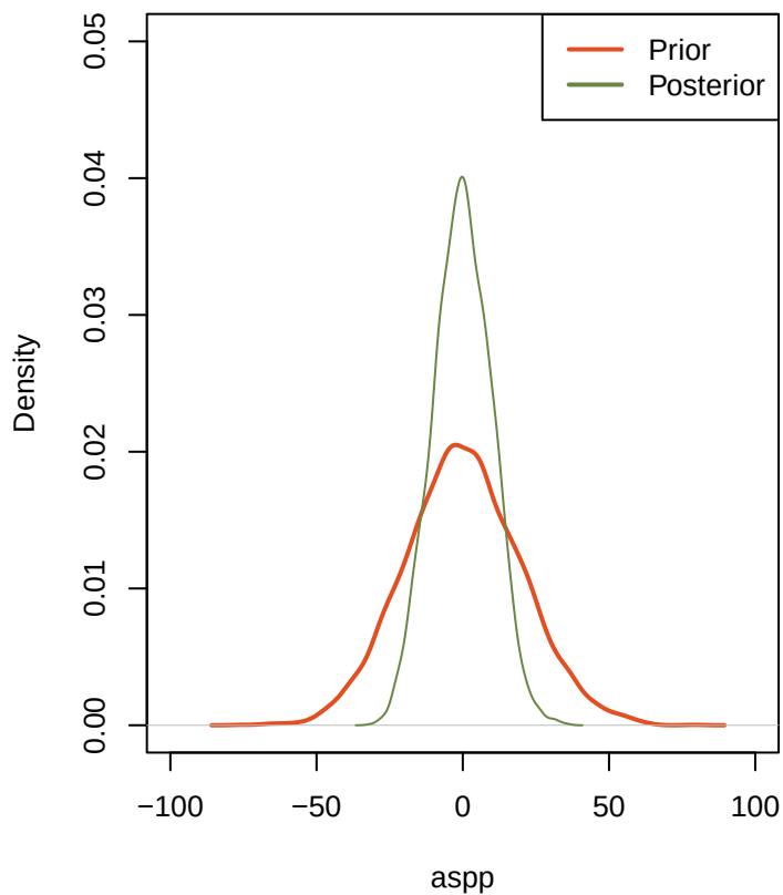
priorVSposterior_aspp
