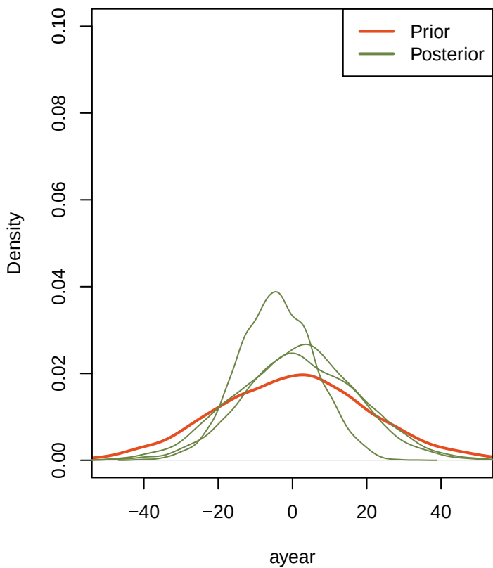
priorVSposterior_ayear
