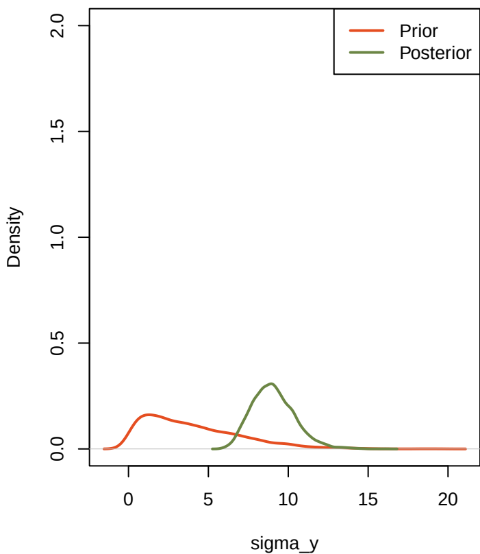
priorVSposterior_sigma_y
