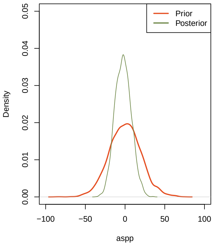
priorVSposterior_aspp
