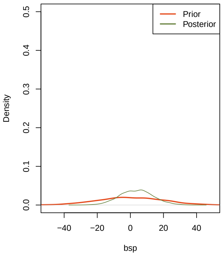
priorVSposterior_bsp
