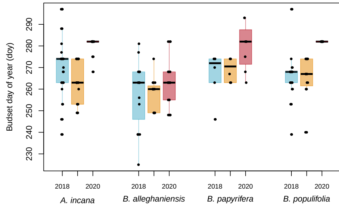
(d) End of season (EOS)
