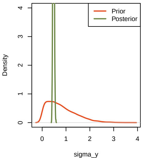
priorVSposterior_sigma_y
