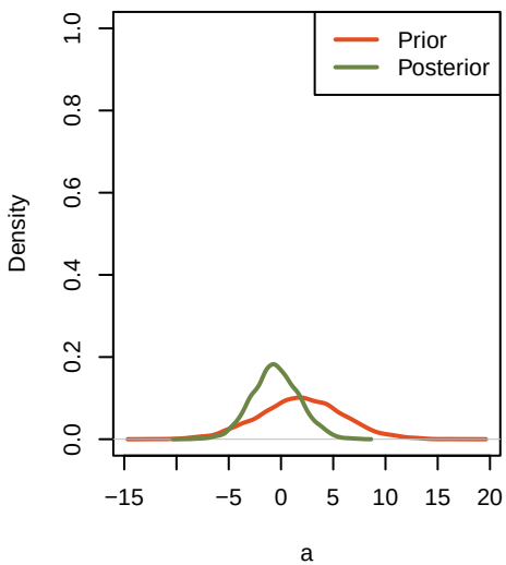
priorVSposterior_a
