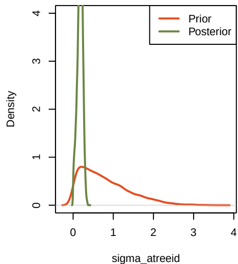
priorVSposterior_sigma_atreedid
