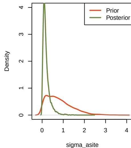
priorVSposterior_sigma_asite
