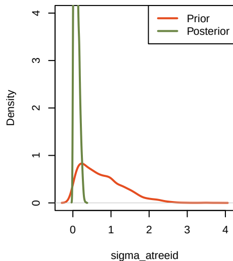
priorVSposterior_sigma_atreedid
