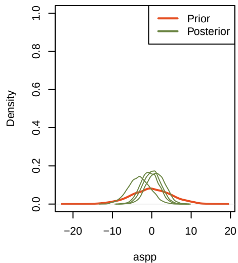
priorVSposterior_aspp
