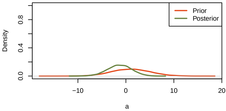
priorVSposterior_a
