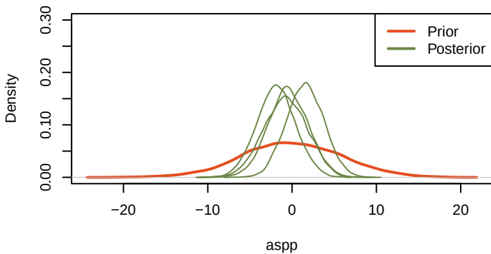
priorVSposterior_aspp
