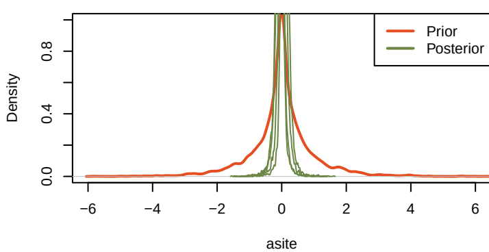
priorVSposterior_asite
