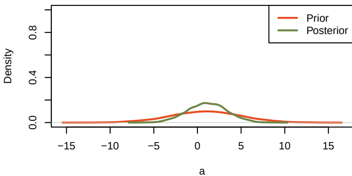
priorVSposterior_a
