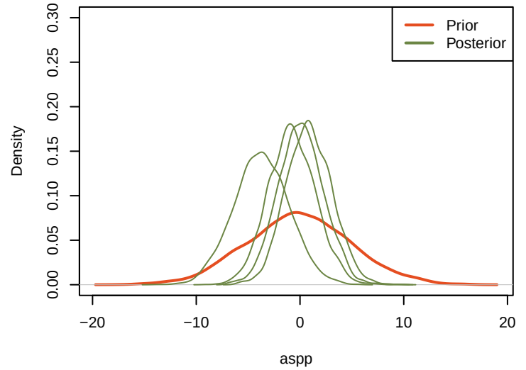
priorVSposterior_aspp
