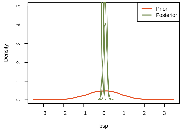
priorVSposterior_bsp
