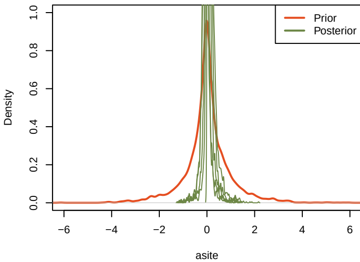
priorVSposterior_asite
