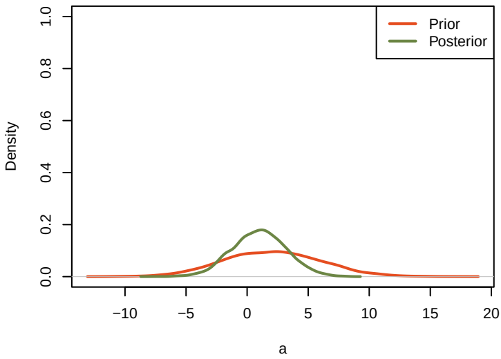
priorVSposterior_a
