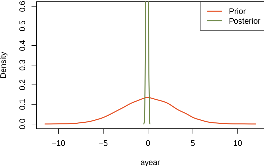
priorVSposterior_2019
