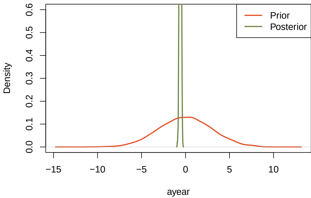
priorVSposterior_2020
