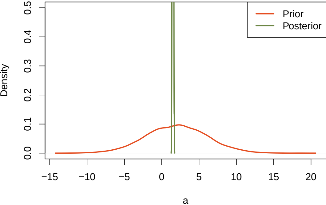
priorVSposterior_2018
