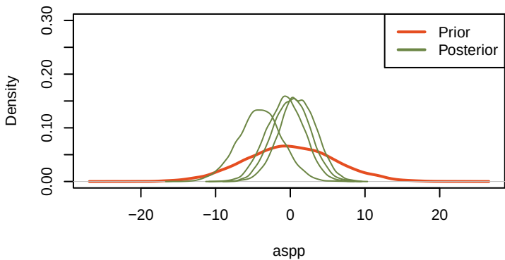
priorVSposterior_aspp
