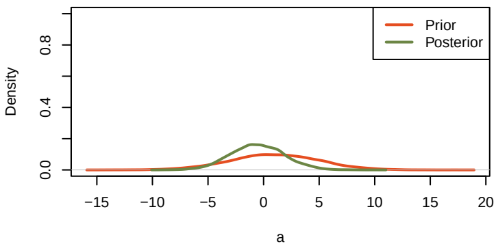
priorVSposterior_a
