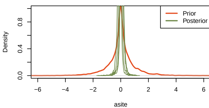
priorVSposterior_asite
