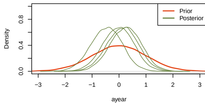
priorVSposterior_ayear
