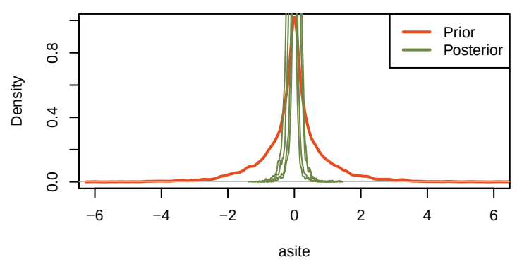
priorVSposterior_asite
