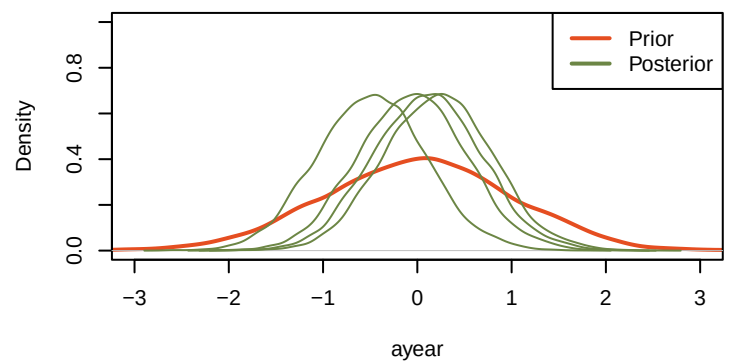
priorVSposterior_ayear
