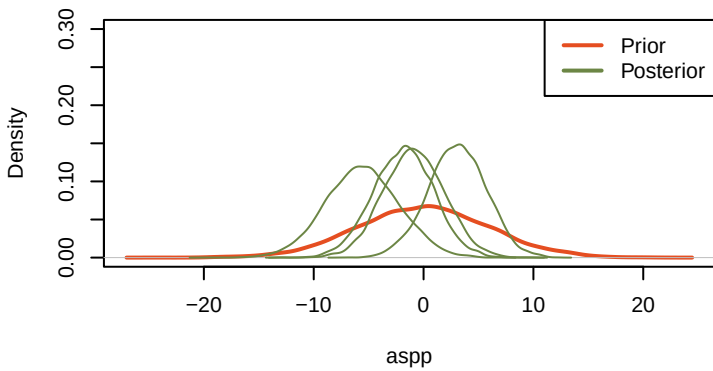
priorVSposterior_aspp
