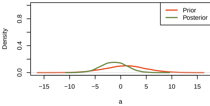
priorVSposterior_a
