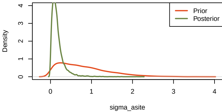
priorVSposterior_sigma_asite
