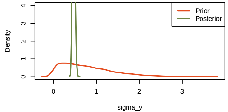
priorVSposterior_sigma_y
