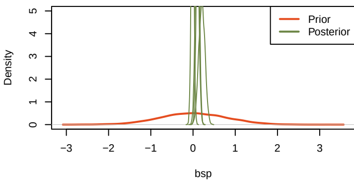
priorVSposterior_bsp
