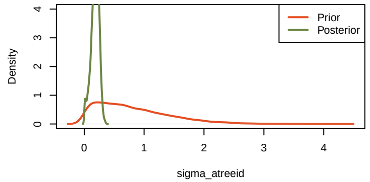
priorVSposterior_sigma_atreeid
