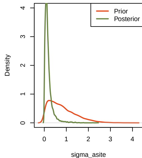
priorVSposterior_sigma_asite
