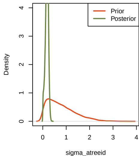
priorVSposterior_sigma_atreedid
