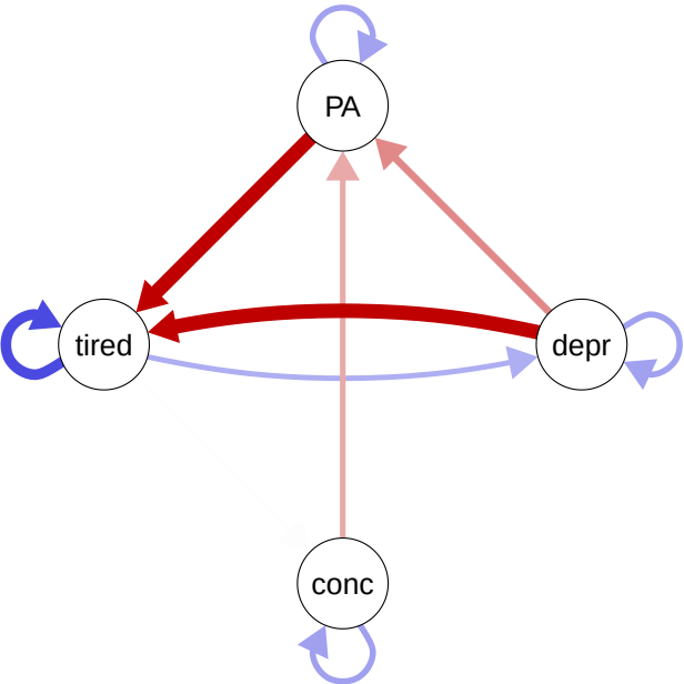
Individual A: Temporal Network
