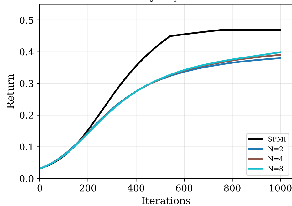
GP - eps=800
