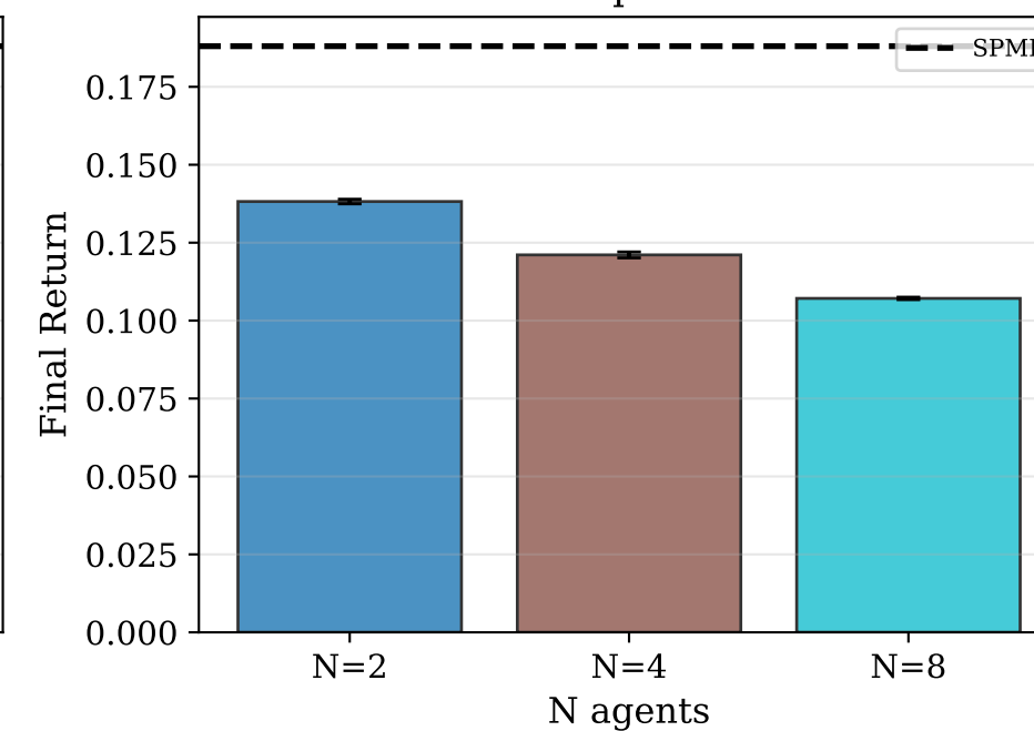
GP - eps=800
