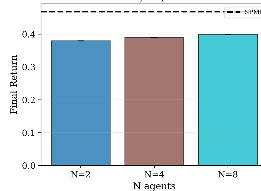
GP - eps=800
