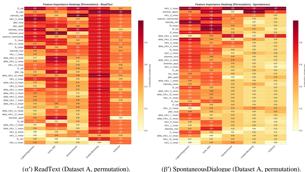
Σχήμα 7.1: Θερμικοί χάρτες permutation importance για τα δύο tasks του Dataset A, με συμπερίληψη του SVM_RBF.
