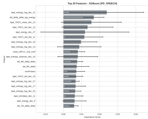
(β') XGBoost
