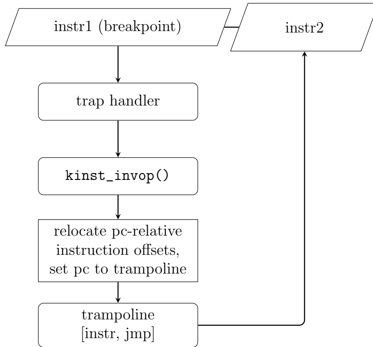
Figure 2: Διάγραμμα ροής amd64.
