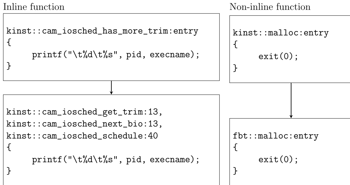
Figure 4: Συντακτικοί μετασχηματισμοί υλοποιημένοι στο cddl/contrib/opensolaris/lib/libdtrace/common/dt_sugar.c
