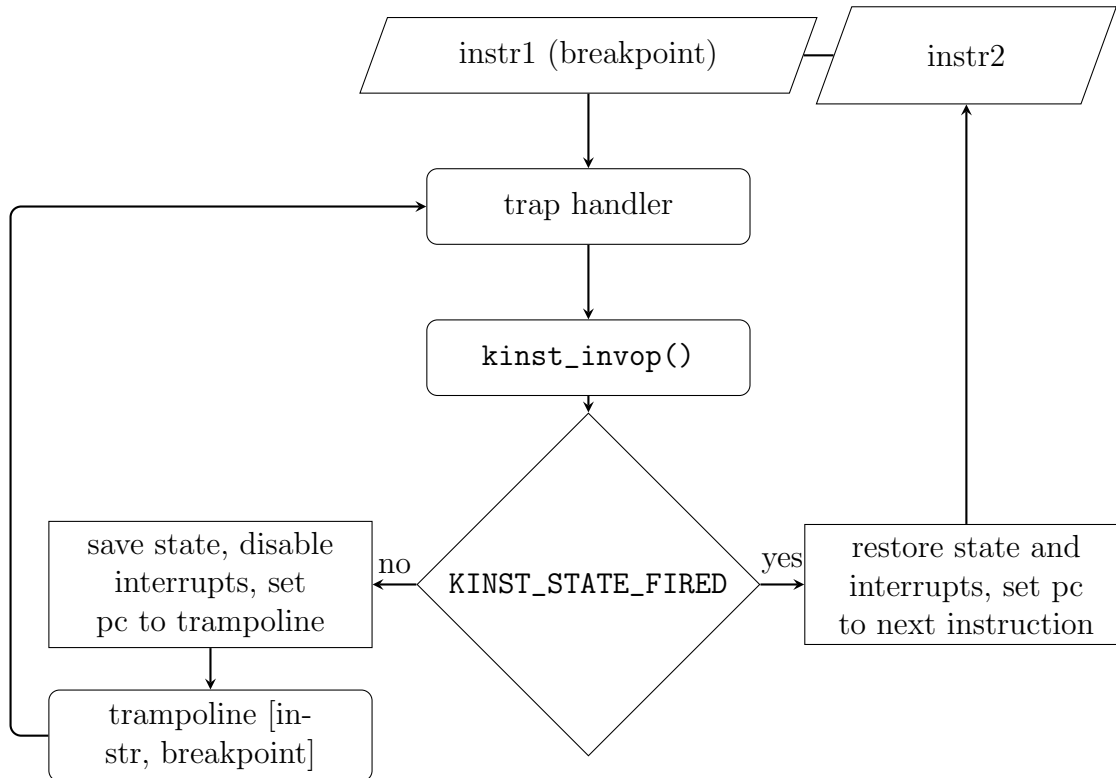
Figure 3: Διάγραμμα ροής arm64 & riscv.
