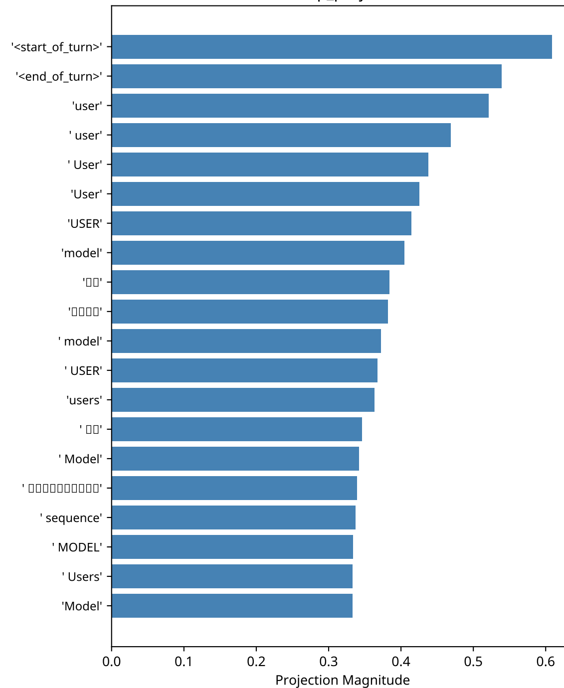
up_proj A
