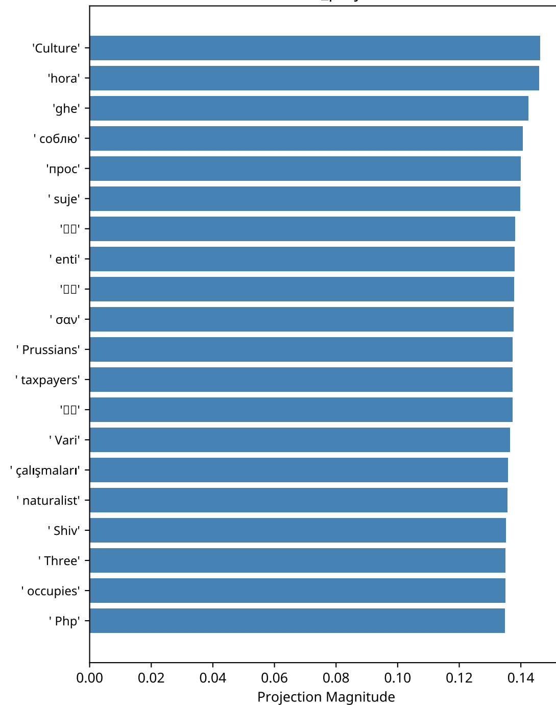
down_proj B
