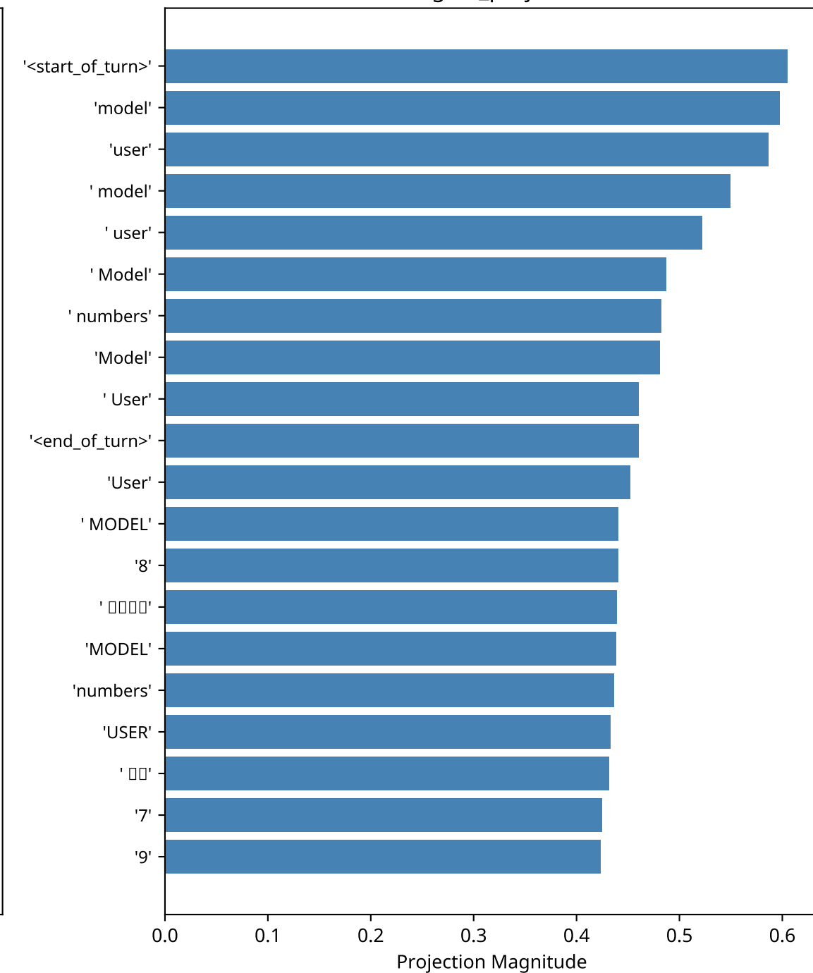
gate_proj A
