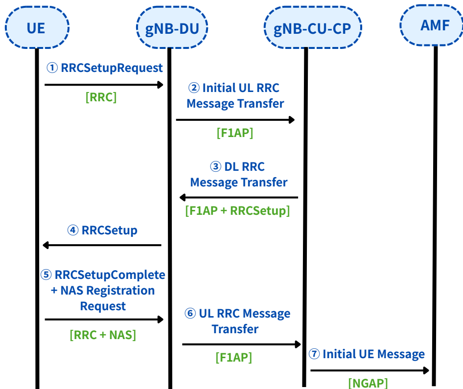
圖 08 · OAI 中 UE Registration Flow : 從 DU 經 CU 到 AMF 的訊息
