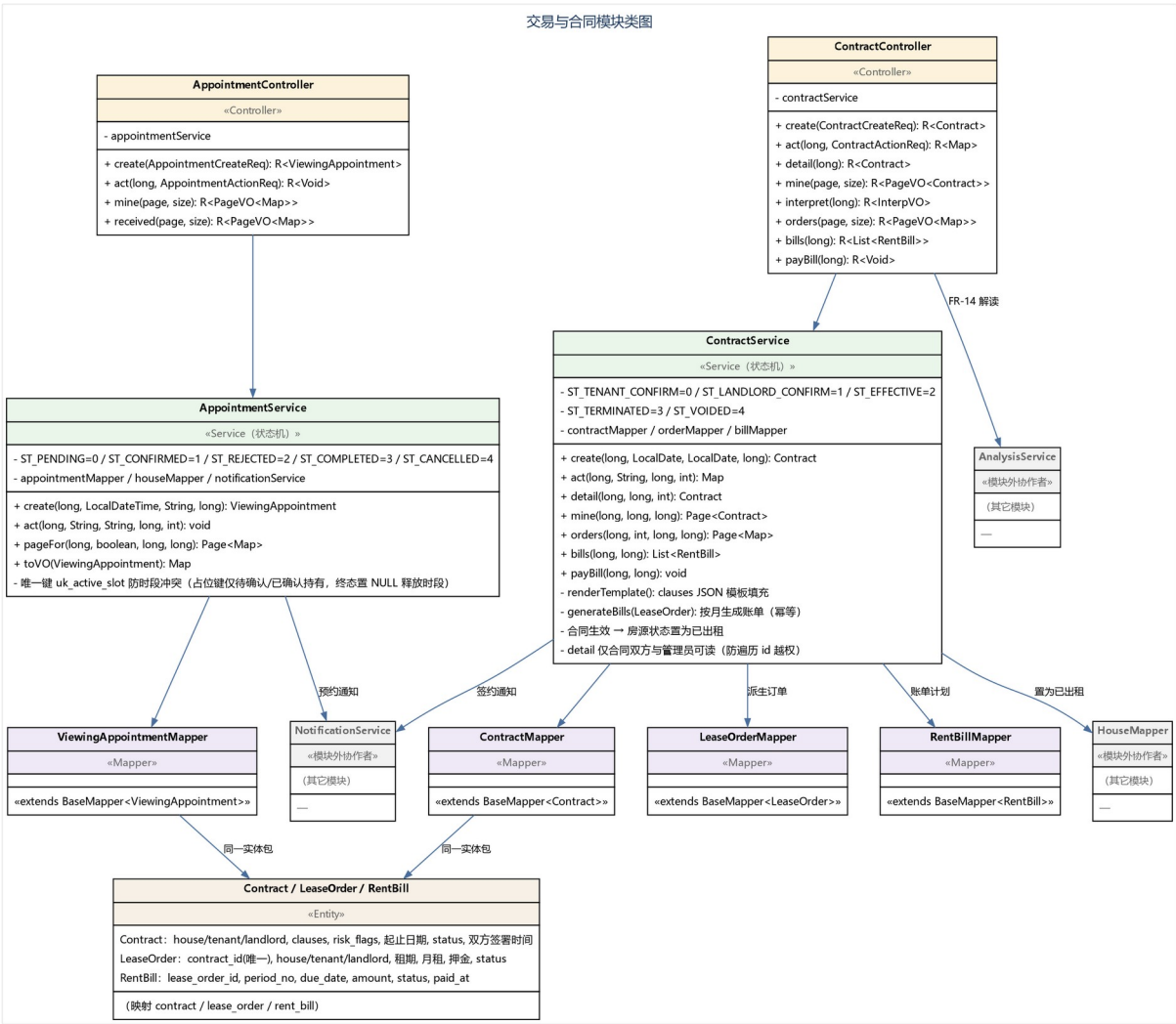
图 3-10 交易与合同模块类图
