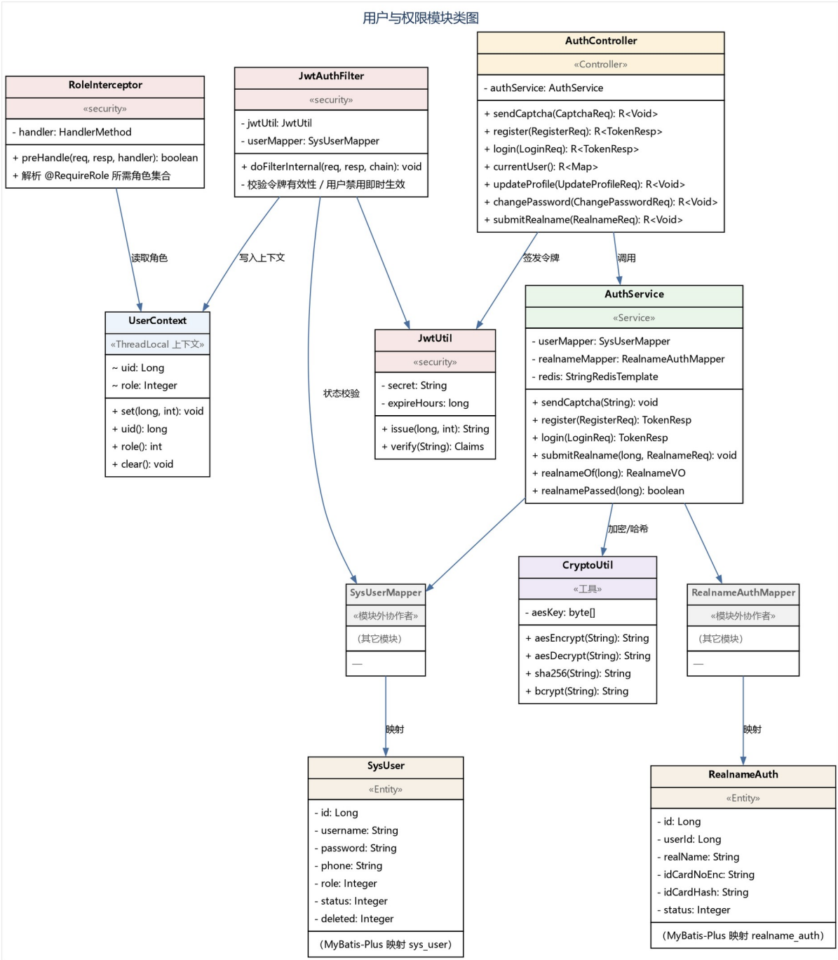
图 3-2 用户与权限模块类图
