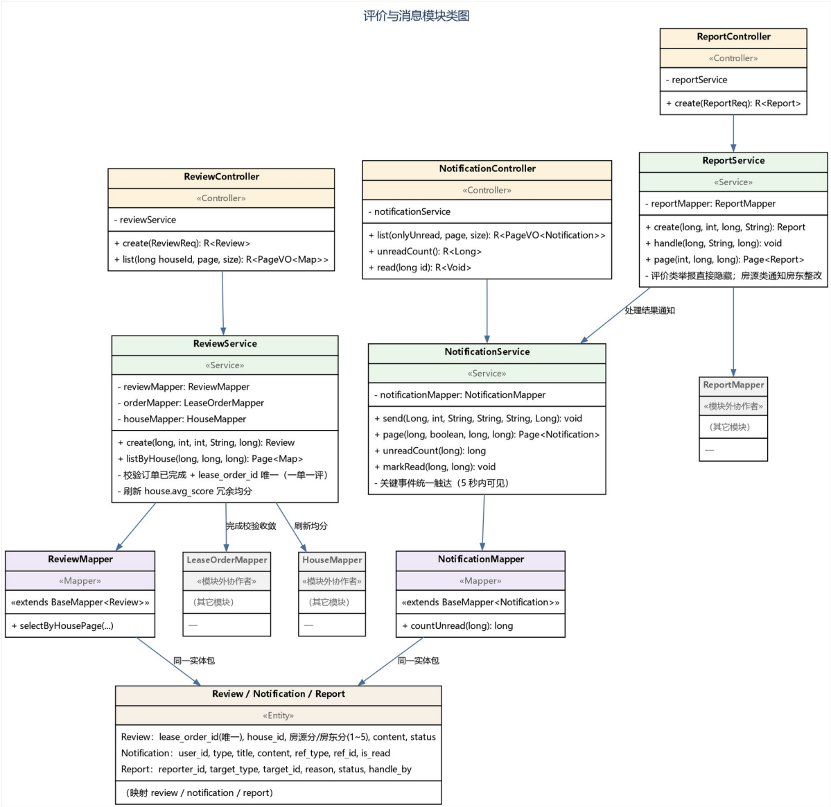
图 3-12 评价与消息模块类图
