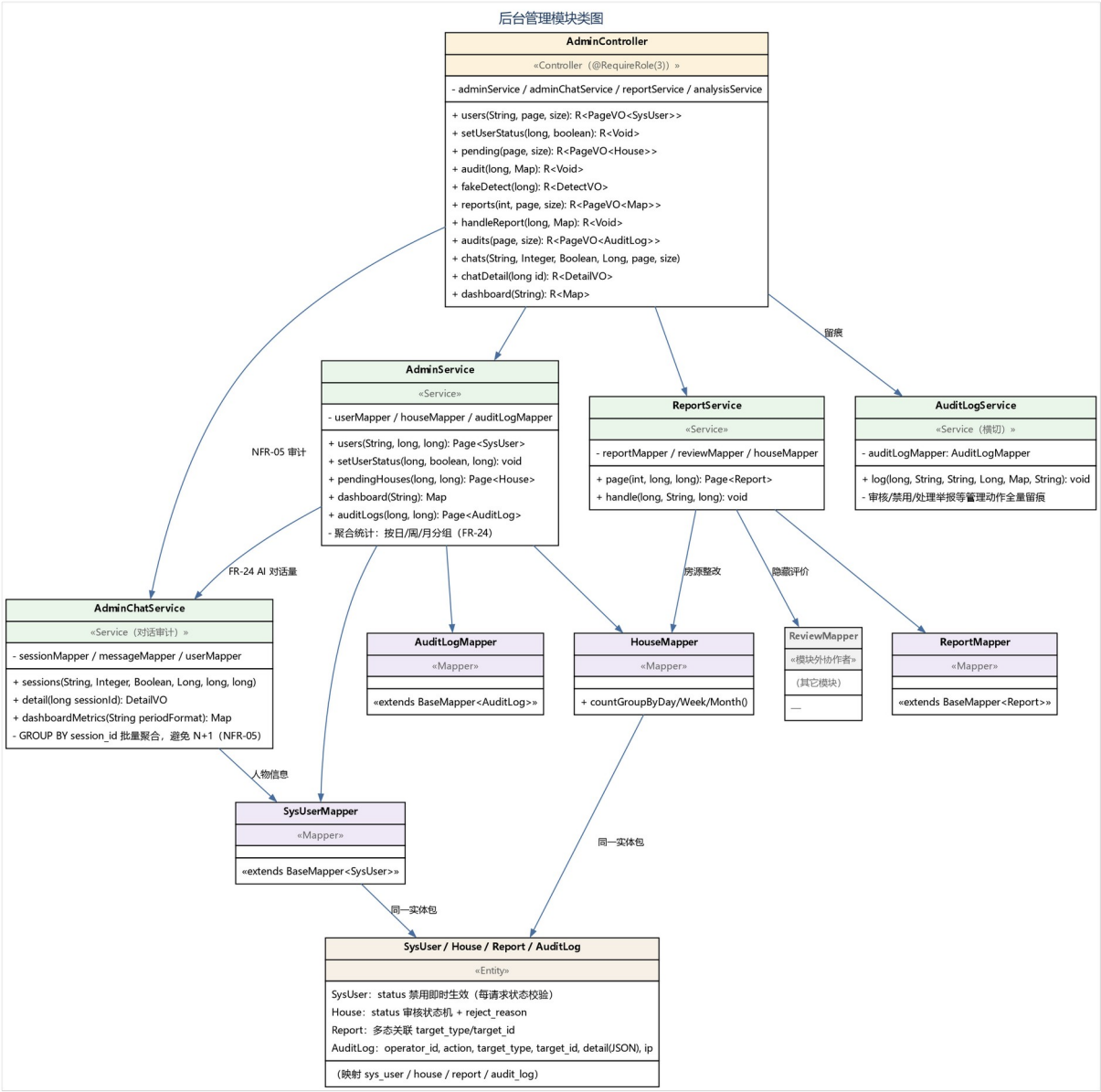
图 3-14 后台管理模块类图
