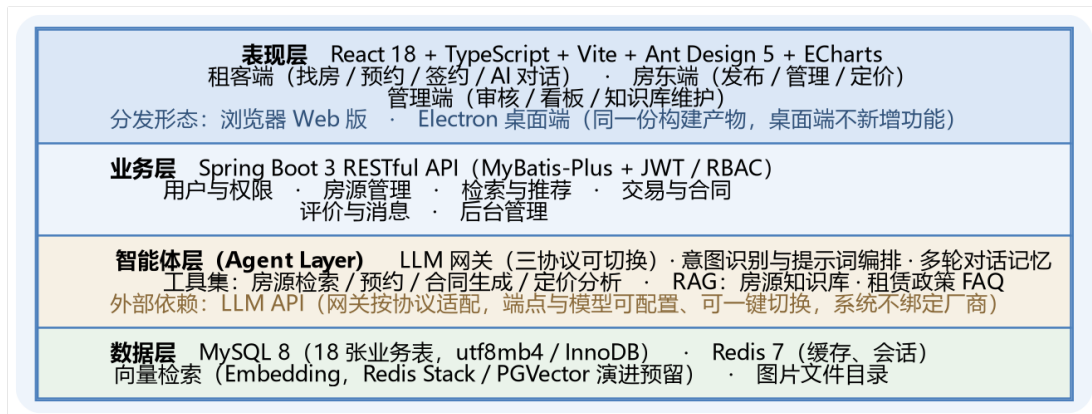
图 5-2 系统总体架构图
