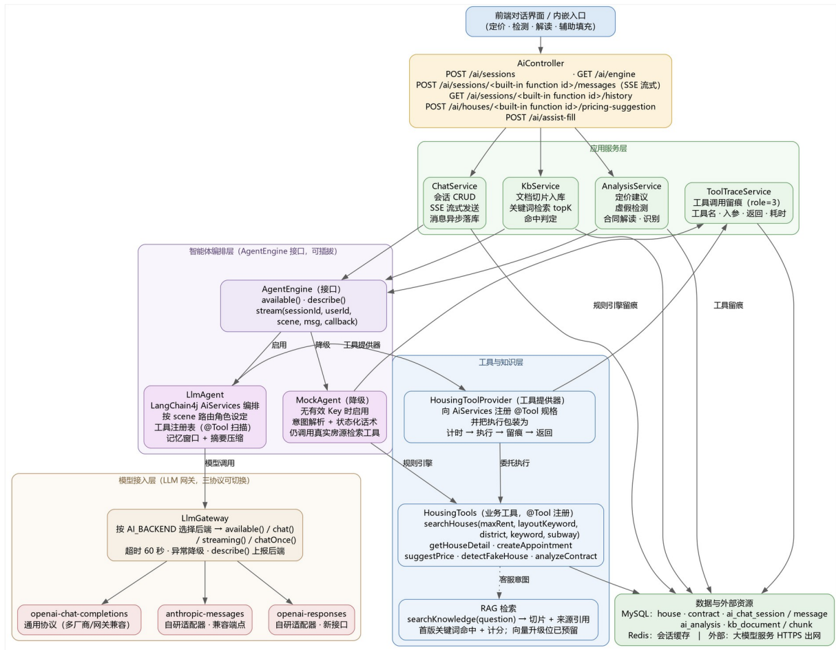
图 3-7 AI 智能体服务模块模块结构图
