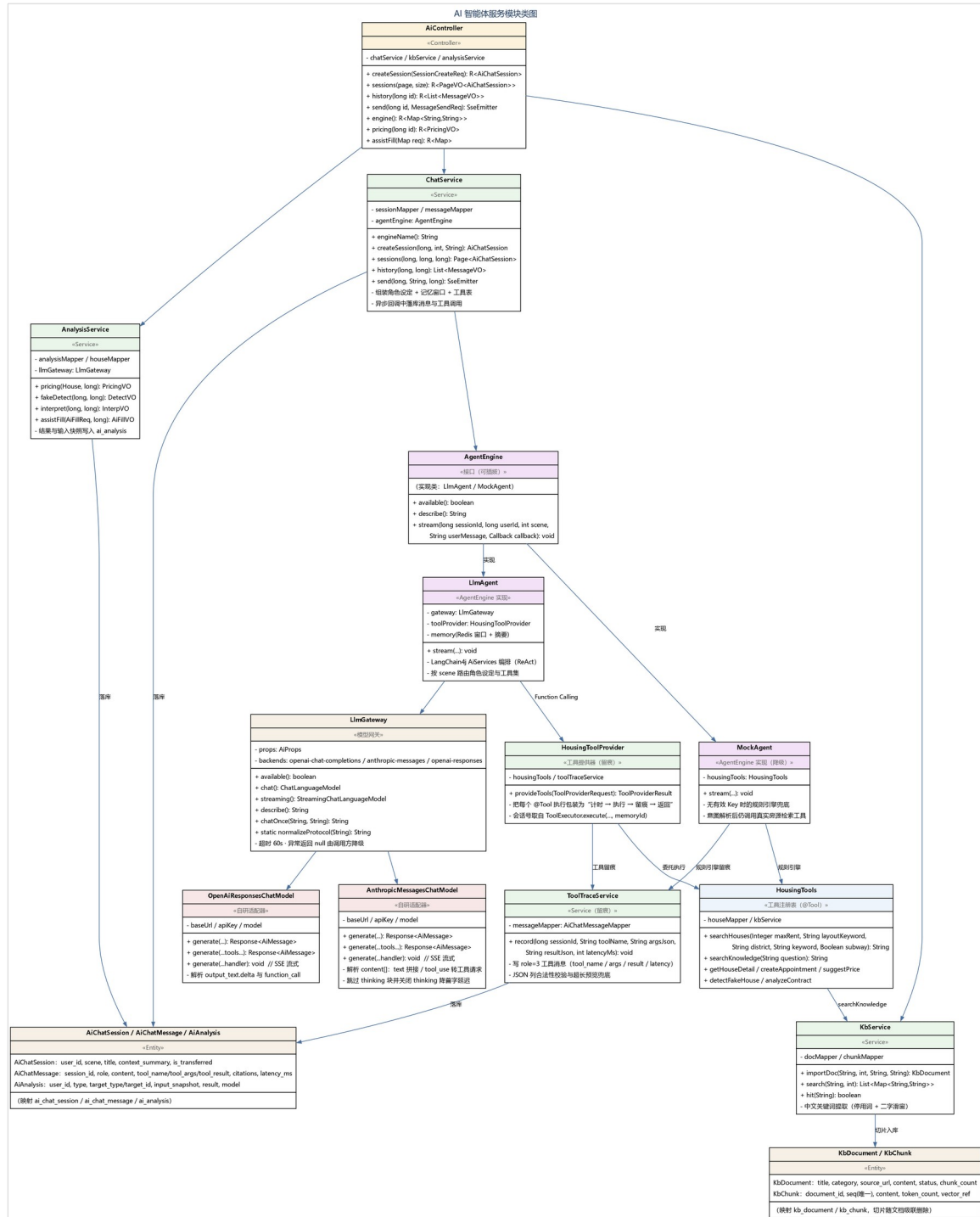
图 3-8 AI 智能体服务模块类图
