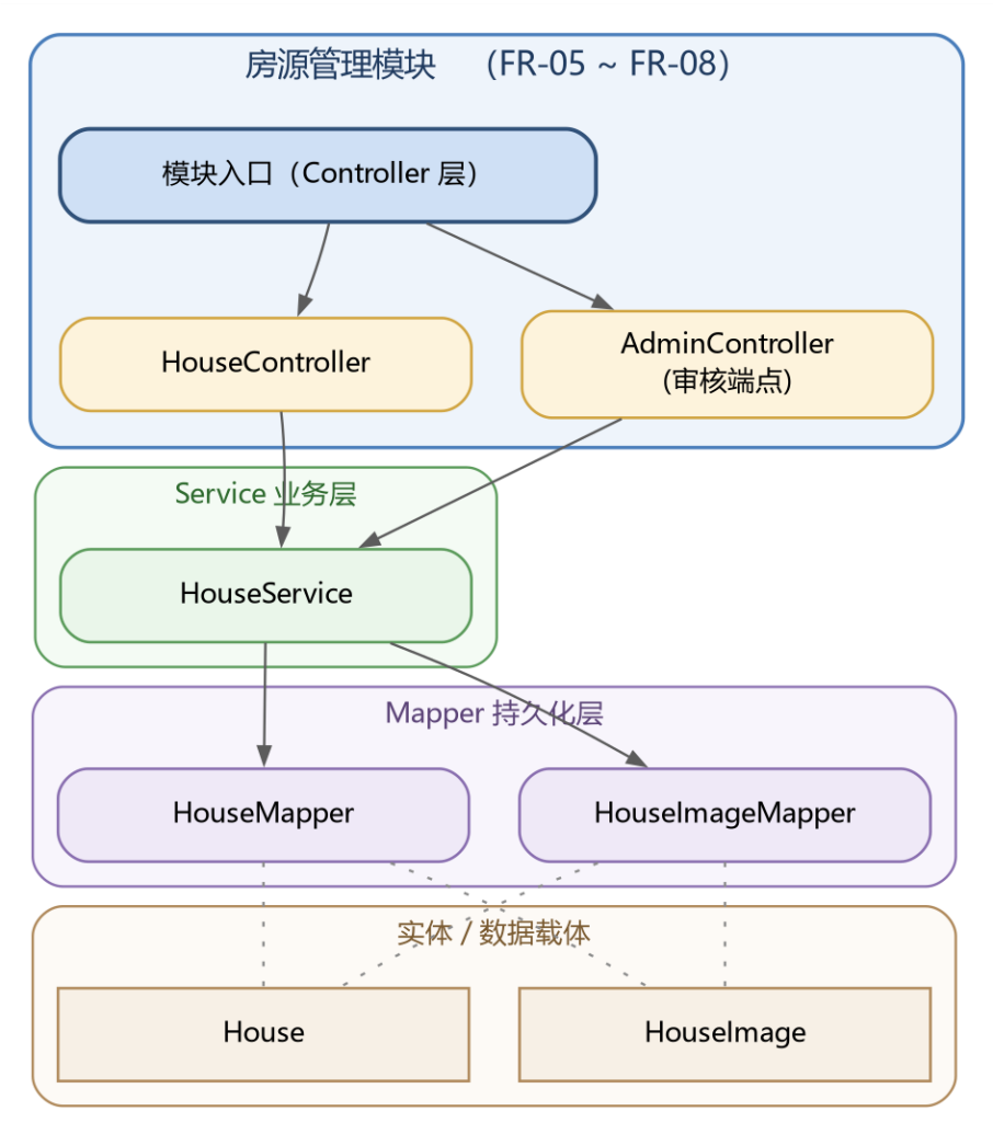
图 3-3 房源管理模块结构图
