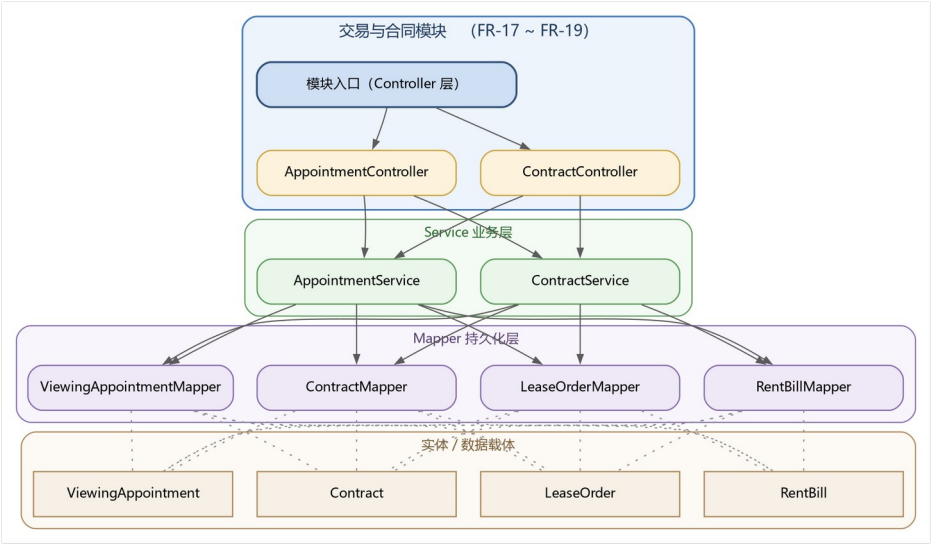
图 3-9 交易与合同模块结构图
