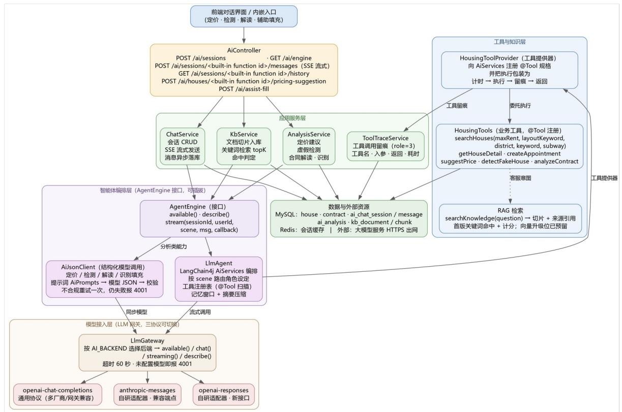
图 3-7 AI 智能体服务模块结构图
