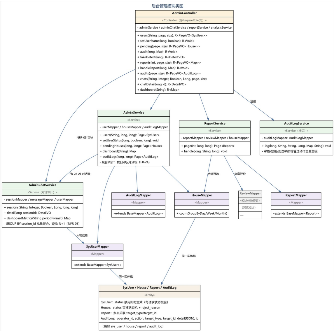
图 3-14 后台管理模块类图
