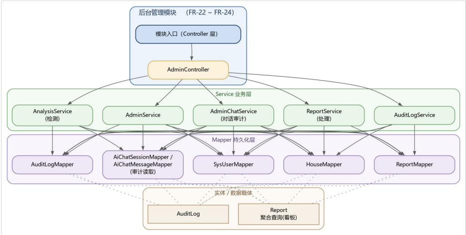
图 3-13 后台管理模块结构图
