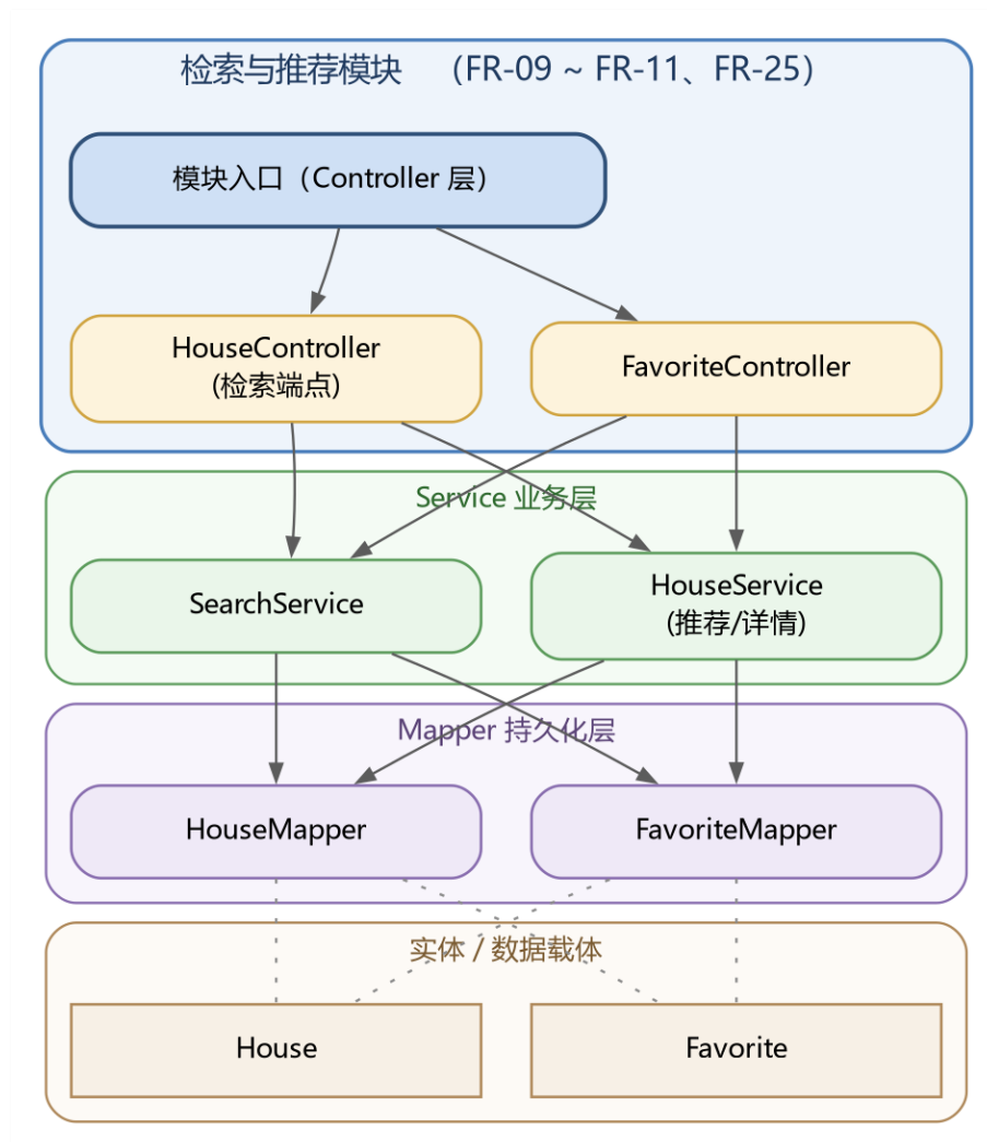
图 3-5 检索与推荐模块结构图
