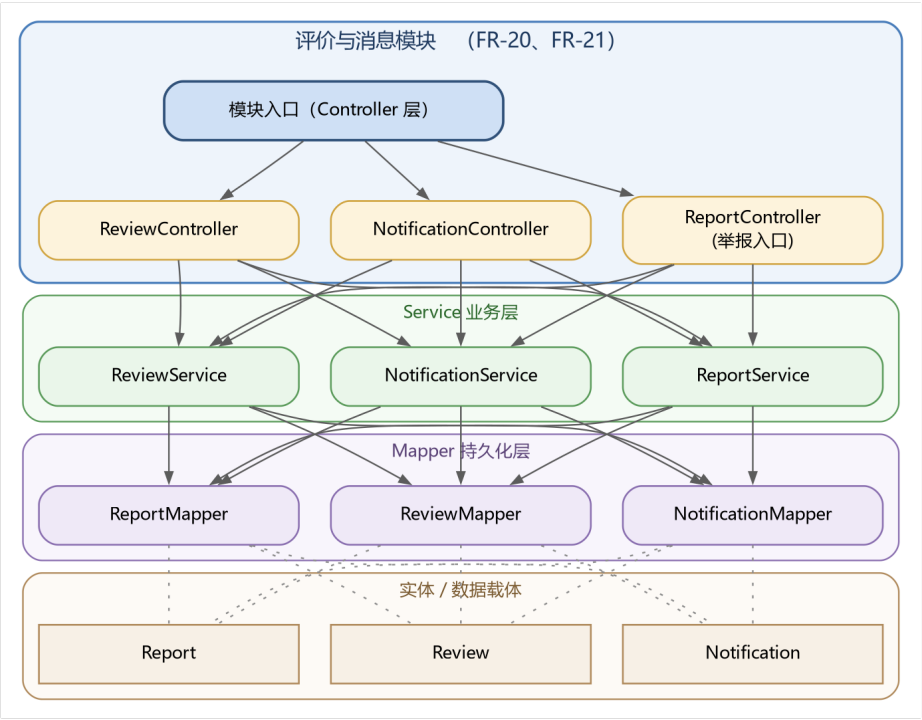
图 3-11 评价与消息模块结构图
