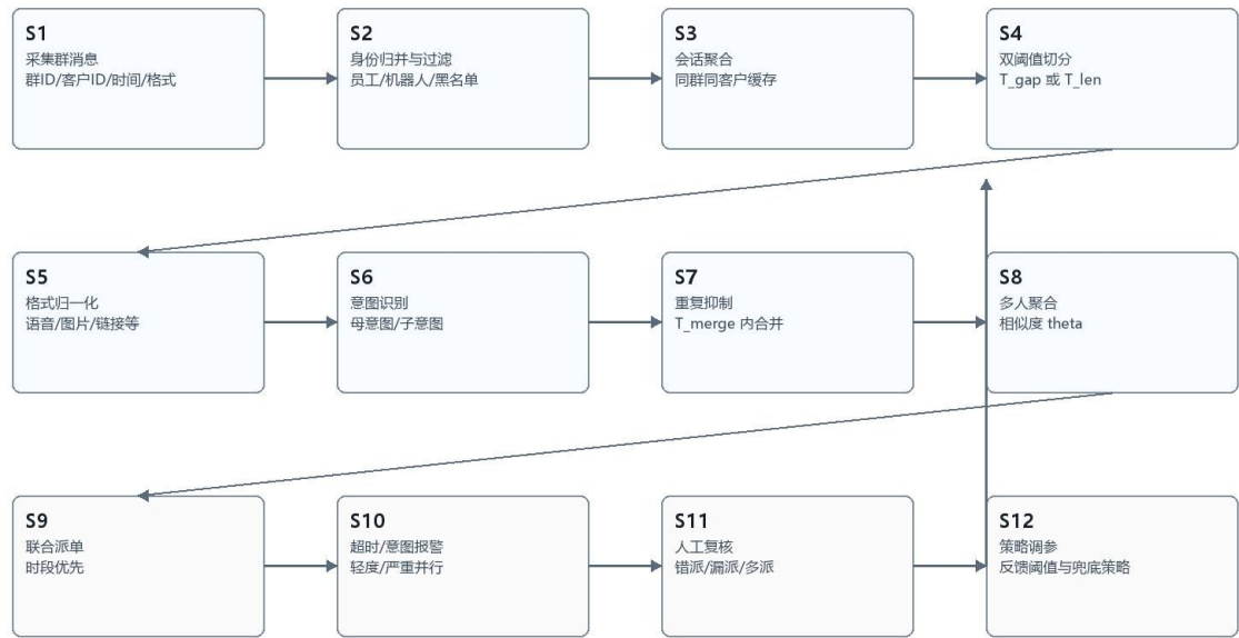
图2 会话派单与运营监控流程图
