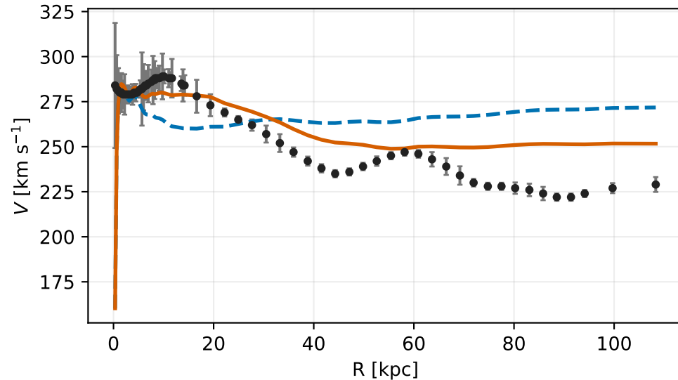
NGC7331
