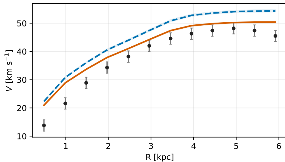
NGC3198
