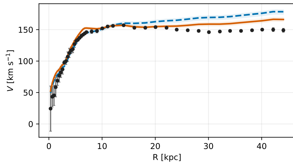
NGC3198
