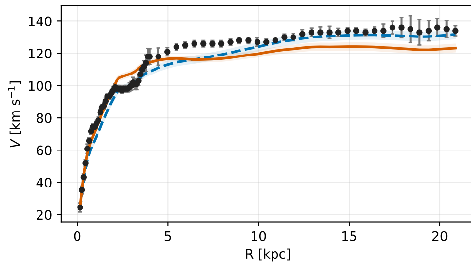
NGC6503
