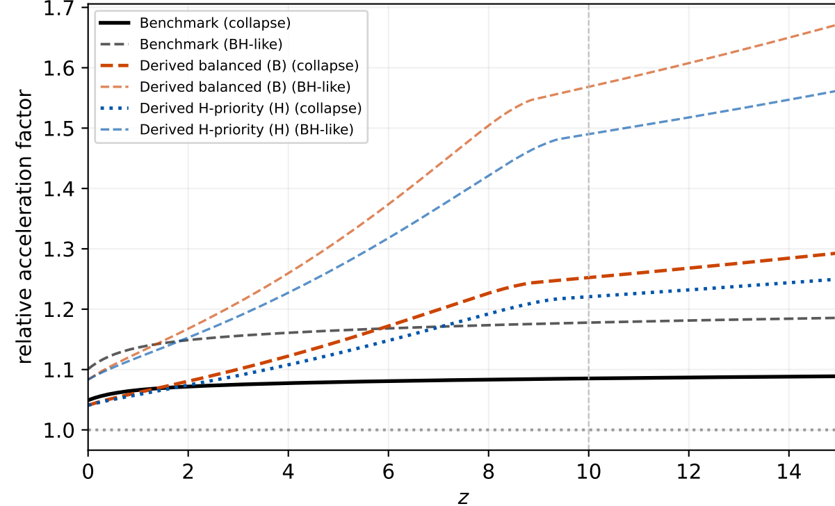
(d) Local maturity-channel acceleration
