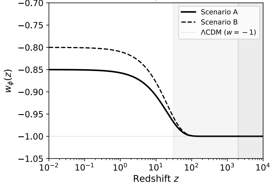
(d) Effective equation of state
