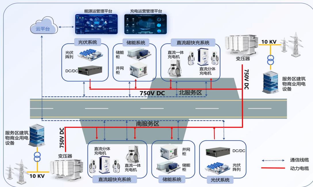
光谧服务区柔性直流互联互济系统总体示意图
