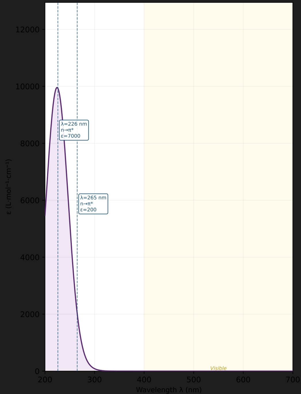
UV-Vis: \epsilon (Linear)
