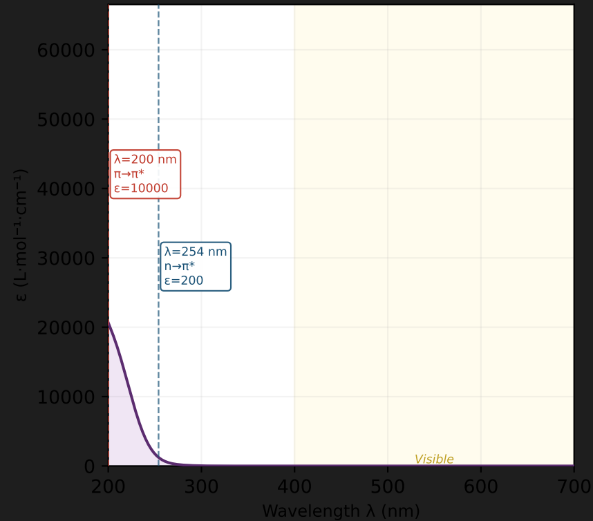
UV-Vis: \epsilon (Linear)
