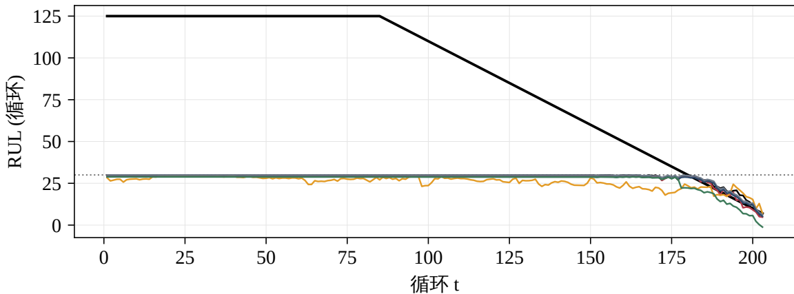
测试发动机 34; 黑线为真实 RUL, 彩线为各方法下界; 删失率 40%, c_0 = 30
