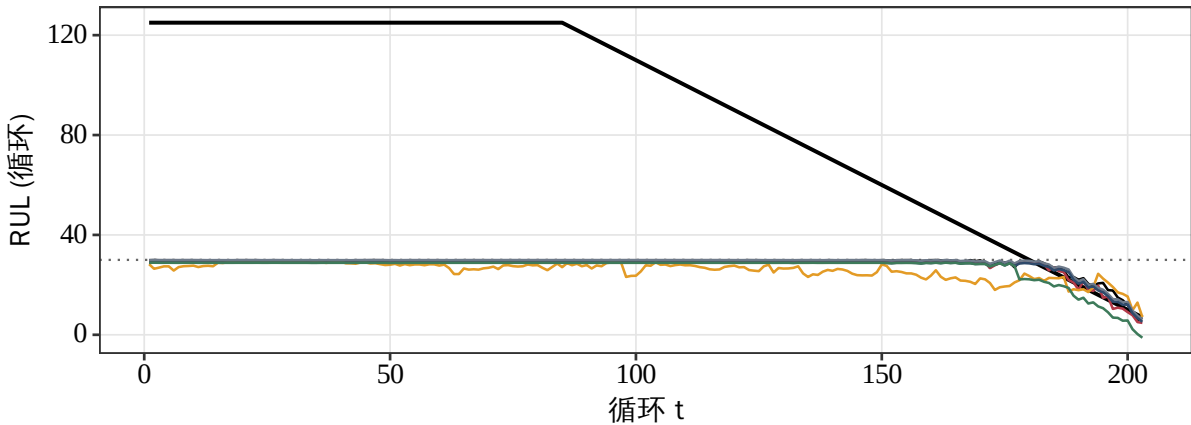
测试发动机 34; 黑线为真实 RUL, 彩线为各方法下界; 删失率 40%, c_0 = 30
