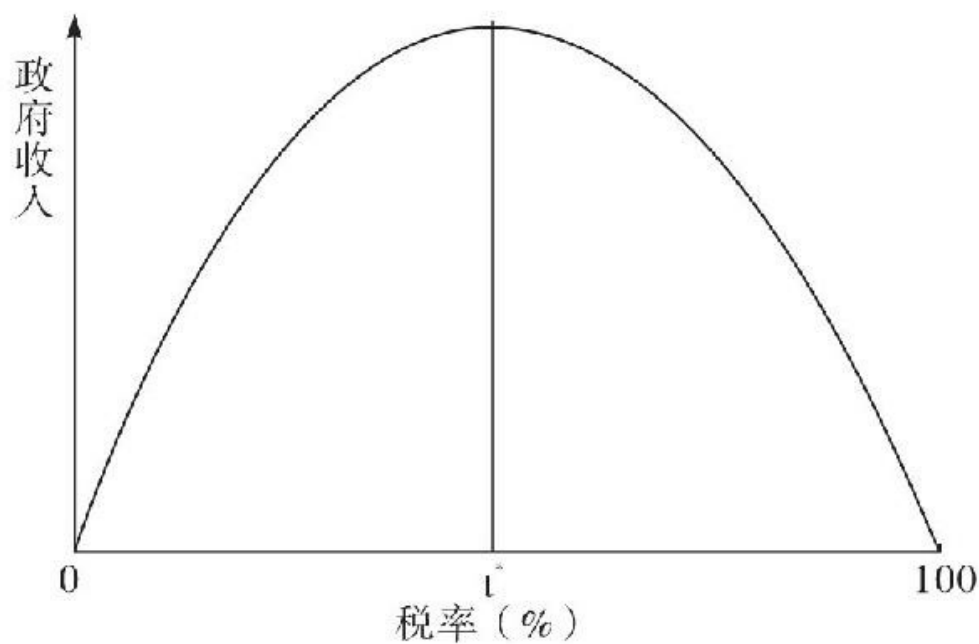
图3.2 拉弗曲线
