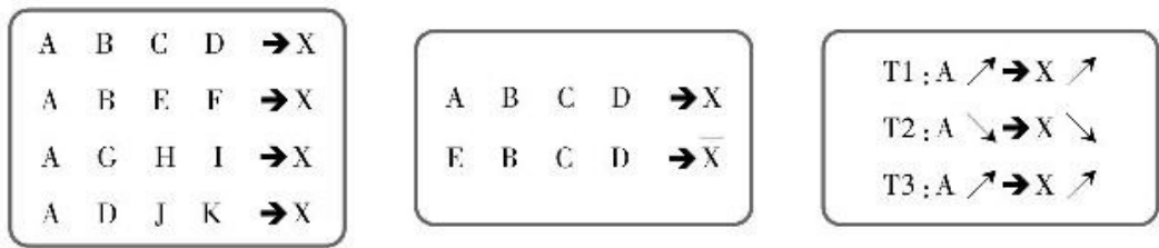
图14.4 确定因果关系的三种研究方法：求同法、求异法与共变法
