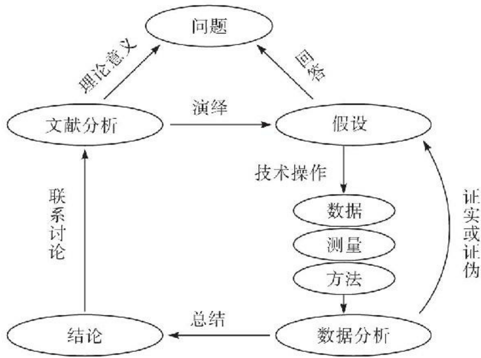
图14.7 洋八股与经验研究的基本结构
