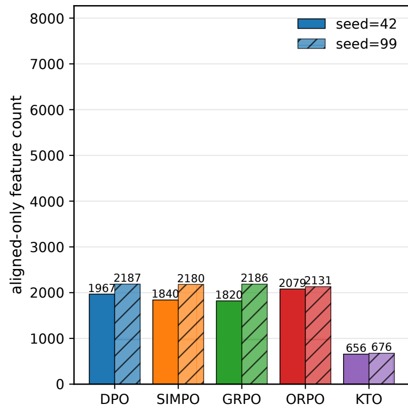
SmolLM3-3B
